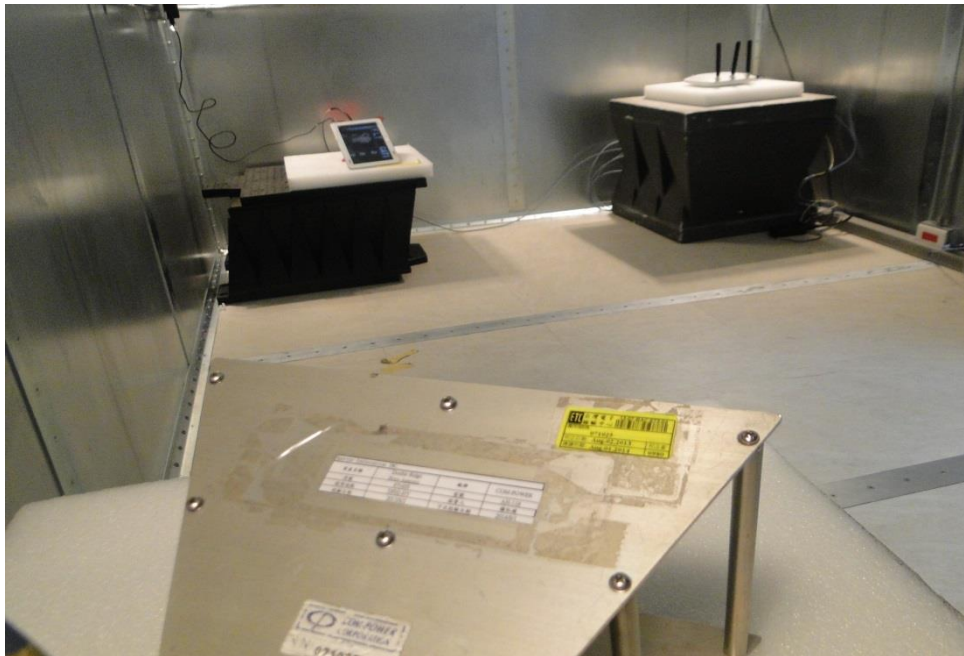
EUT
