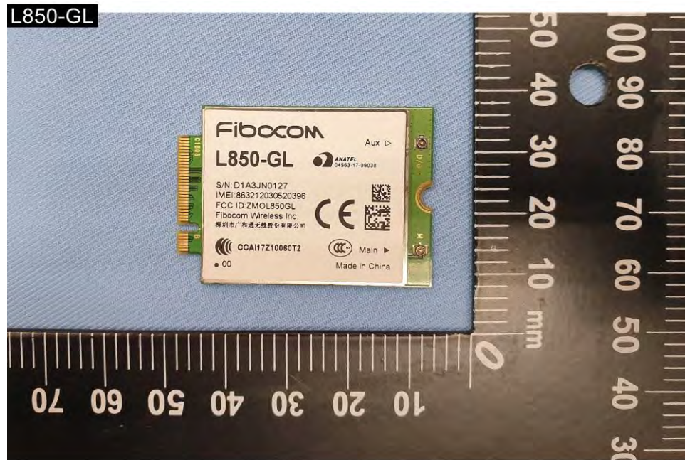
EUT Photo (2)
