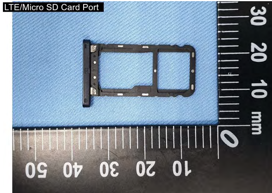
EUT Photo (14)
