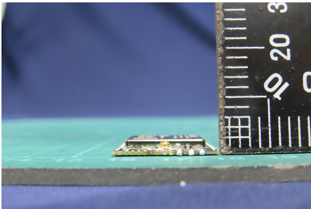
(6) EUT Photo
