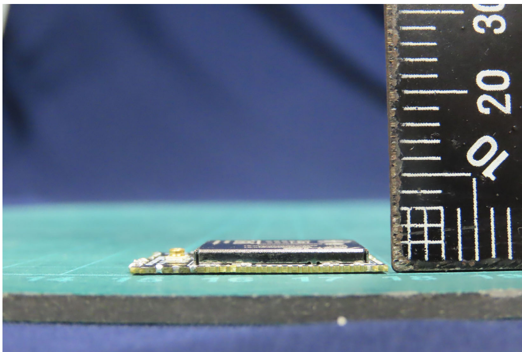
(5) EUT Photo
