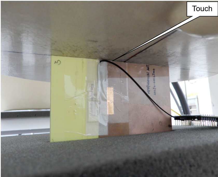
EUT Right-Side
