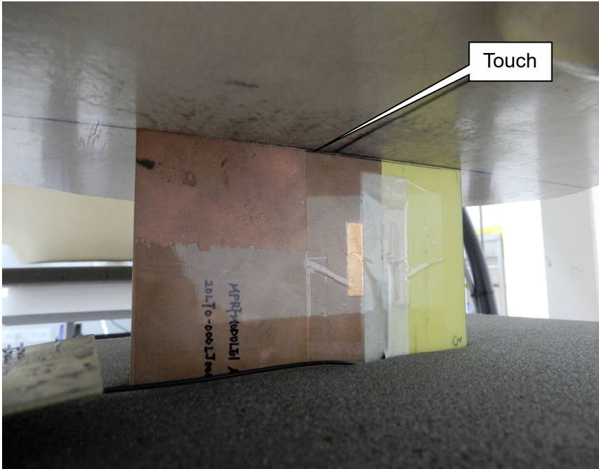
EUT Left-Side
