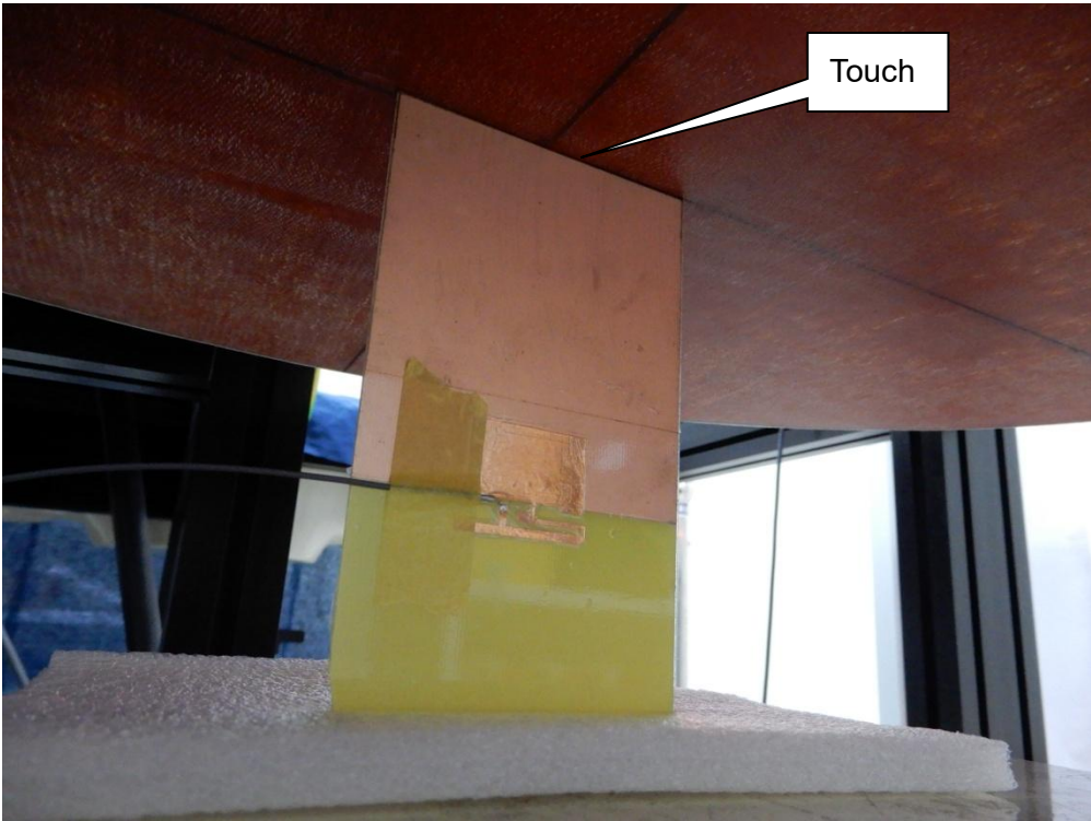
EUT Top
