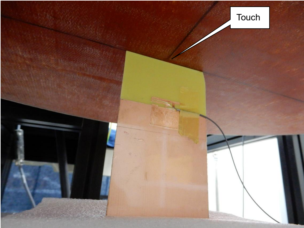
EUT Bottom
