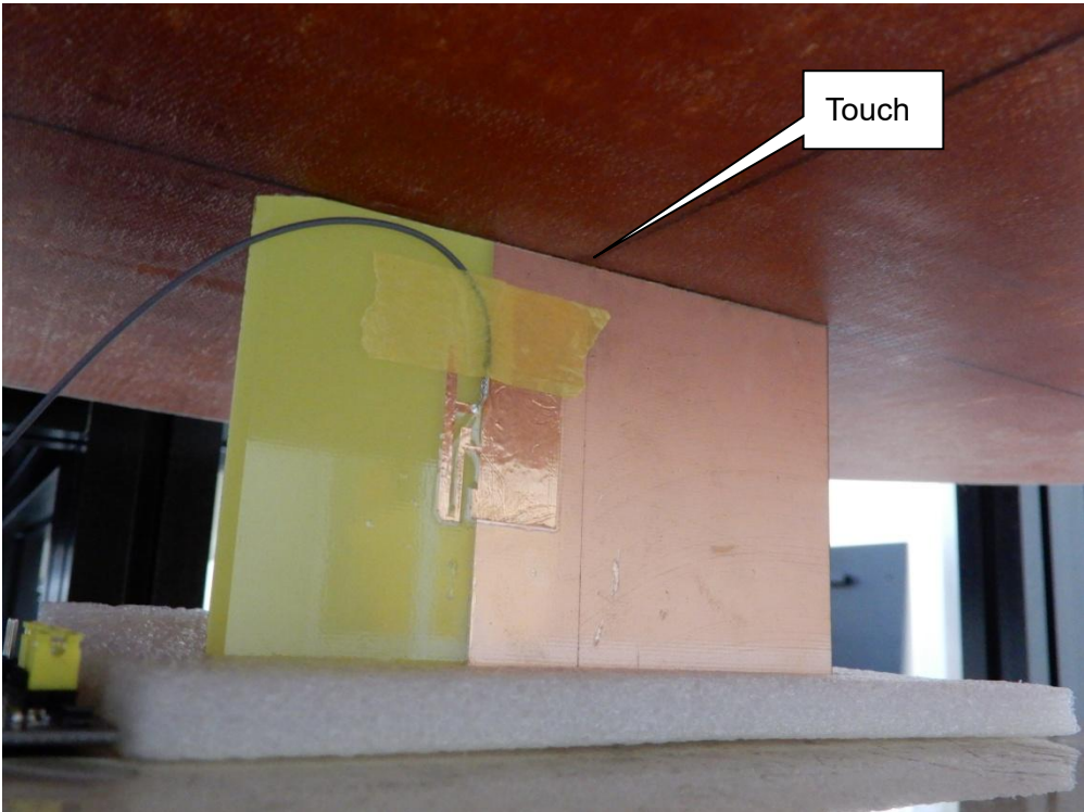
EUT Left-side
