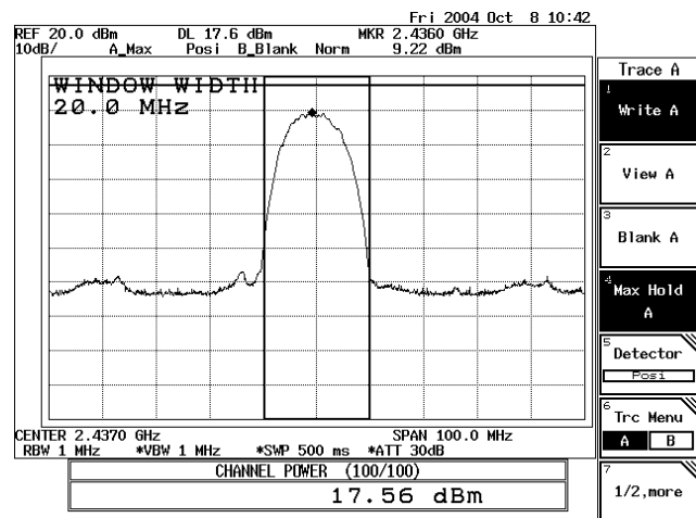
11Mbps-CH 06
