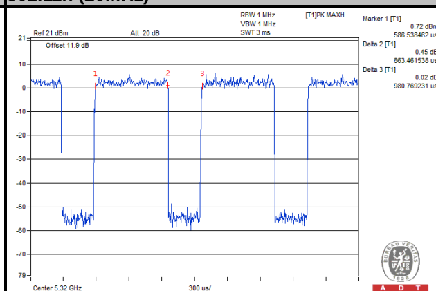
802.11n (20MHz)
