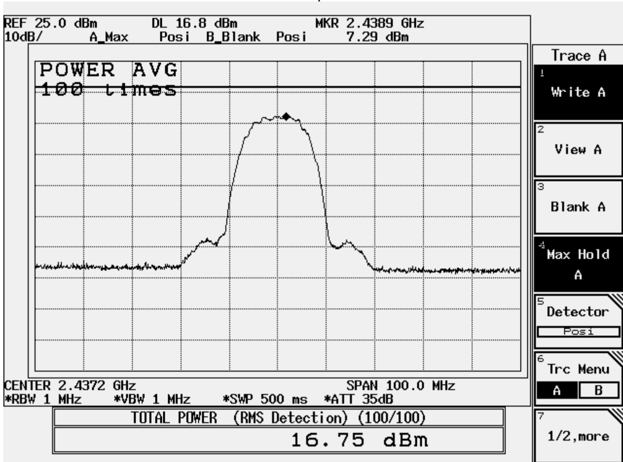
11Mbps-Ch06
