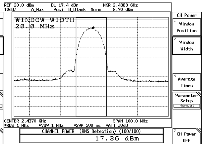
11Mbps-CH 06
