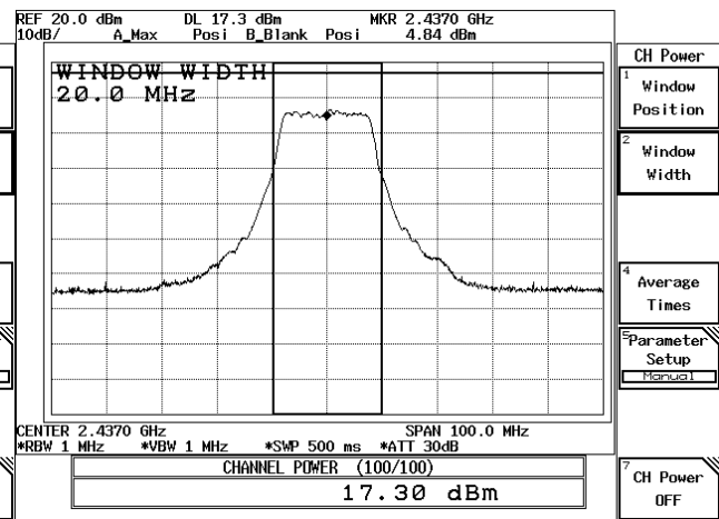
54Mbps-CH 06
