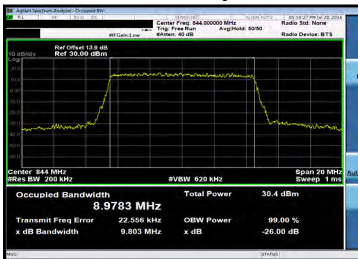
Band26 10MHz_QPSK 50 0_HighCH26990-844
