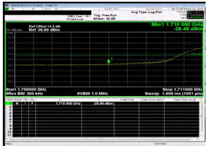
Band Edge_Band4 20MHz_QPSK 100 0_LowCH20050-1720
