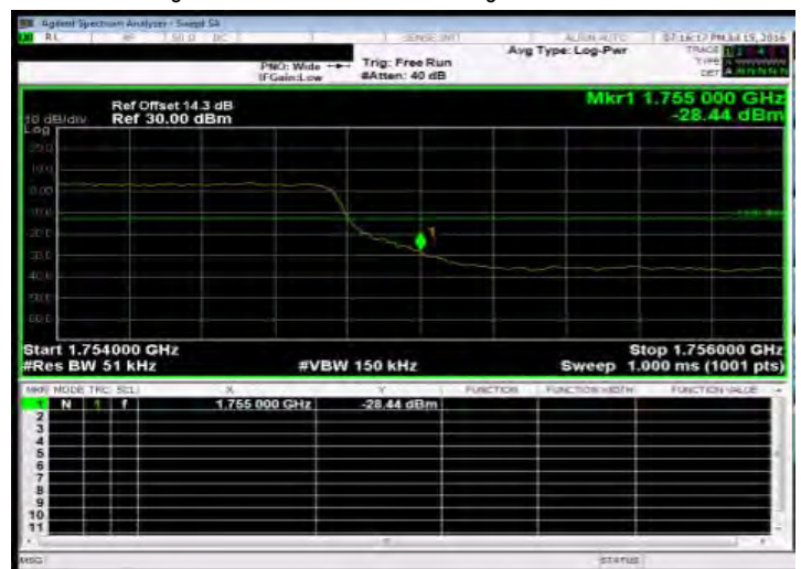
Band Edge_Band4 5MHz_QPSK 25 0_HighCH20375-1752.5
