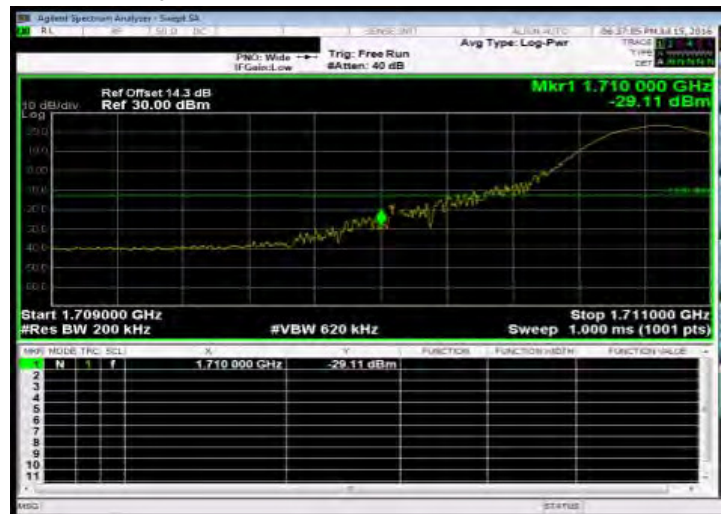
Band Edge_Band4 15MHz_QPSK 1 0_LowCH20025-1717.5
