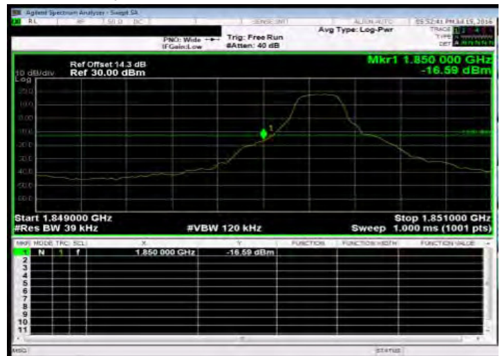
Band Edge_Band2 3MHz_QPSK 1 0_LowCH18615-1851.5
