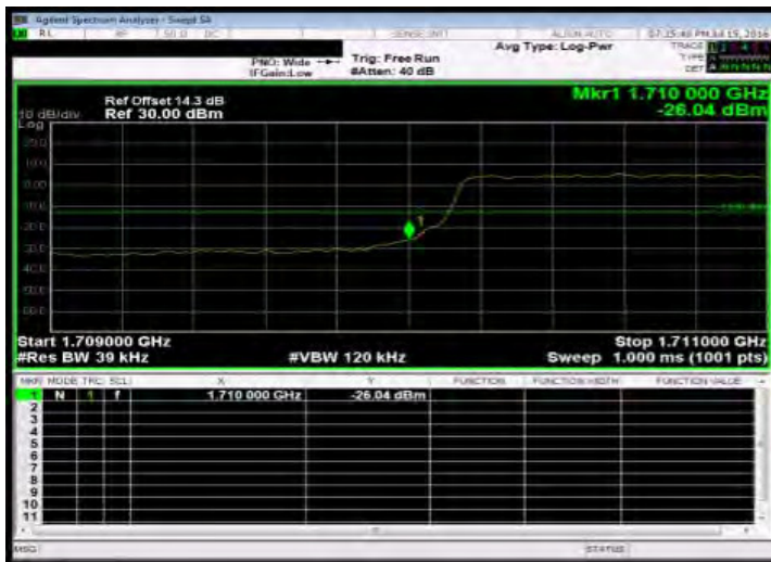
Band Edge_Band4 3MHz_QPSK 15 0_LowCH19965-1711.5
