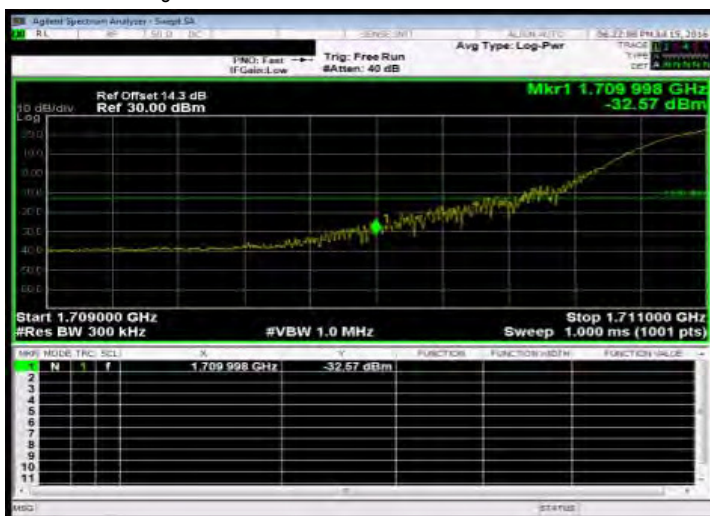
Band Edge_Band4 20MHz_QPSK 1 0_LowCH20050-1720
