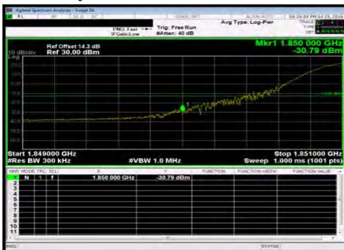
Band Edge_Band2 20MHz_QPSK 1 0_LowCH18700-1860
