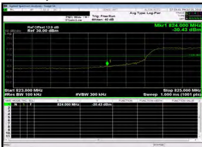
Band Edge_Band5 10MHz_QPSK 50 0_LowCH20450-829
