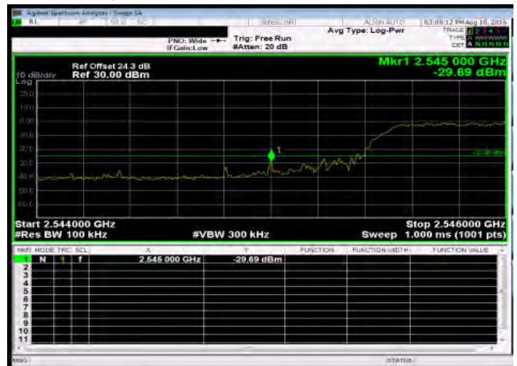
Band Edge_Band41 10MHz_QPSK 50 0_LowCH40190-2550
