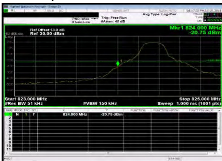
Band Edge_Band5 5MHz_QPSK 1 0_LowCH20425-826.5
