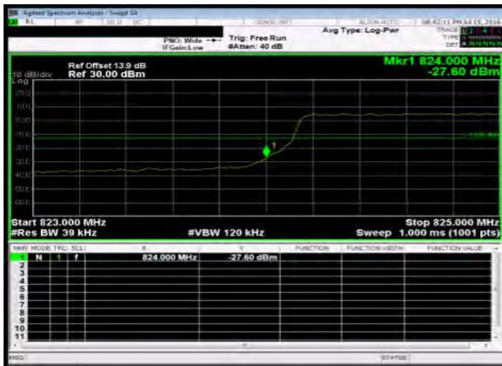
Band Edge_Band5 3MHz_QPSK 15 0_LowCH20415-825.5
