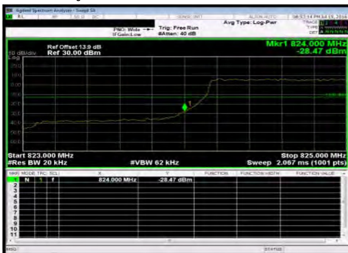
Band Edge_Band5 1.4MHz_QPSK 6 0_LowCH20407-824.7
