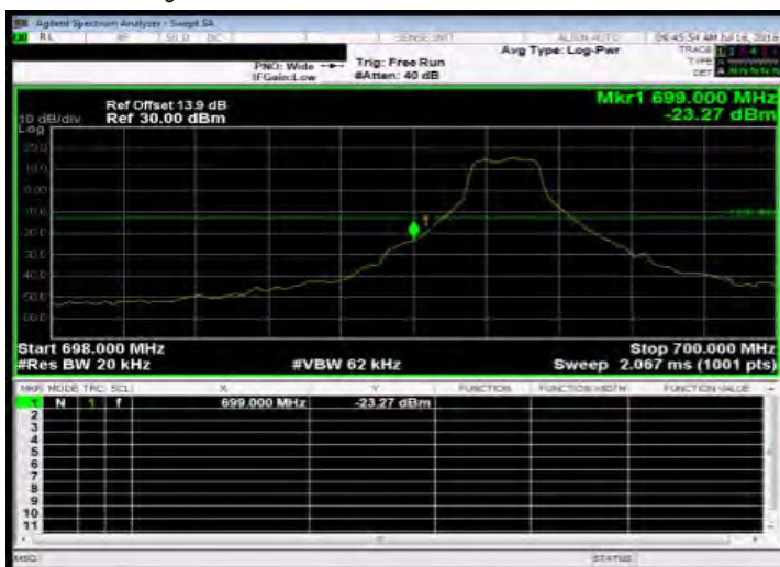
Band Edge_Band12 1.4MHz_QPSK 1 0_LowCH23017-699.7
