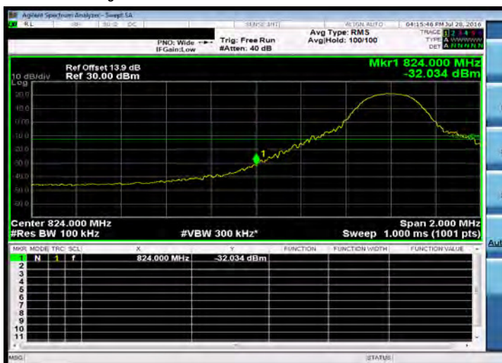
Band Edge_Band26 10MHz_QPSK 1 0_LowCH26840-829.0
