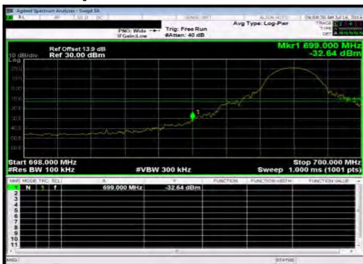
Band Edge_Band12 10MHz_QPSK 1 0_LowCH23060-704
