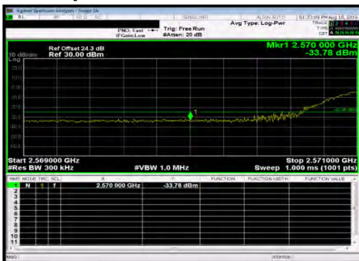
Band Edge_Band38 20MHz_QPSK 100 0_LowCH37850-2580
