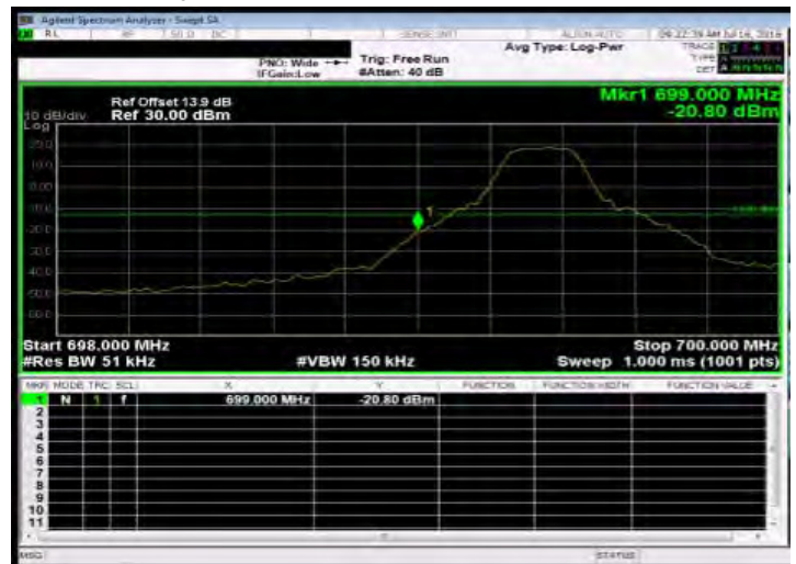
Band Edge_Band12 5MHz_QPSK 1 0_LowCH23035-701.5
