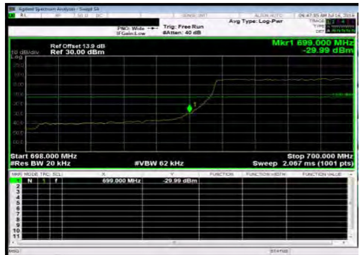
Band Edge_Band12 1.4MHz_QPSK 6 0_LowCH23017-699.7
