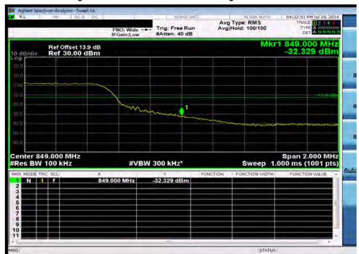
Band Edge_Band26 10MHz_QPSK 50 0_HighCH26990-844
