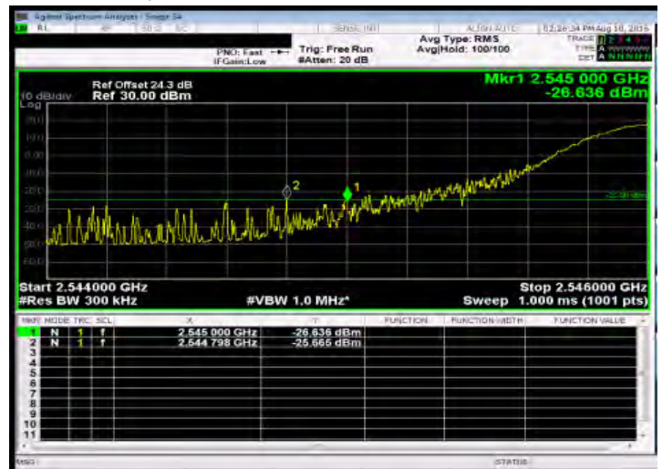
Band Edge_Band41 20MHz_QPSK 1 0_LowCH40240-2555
