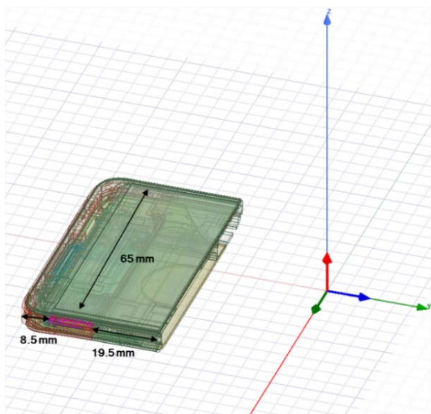
Figure C-6 Bottom module
