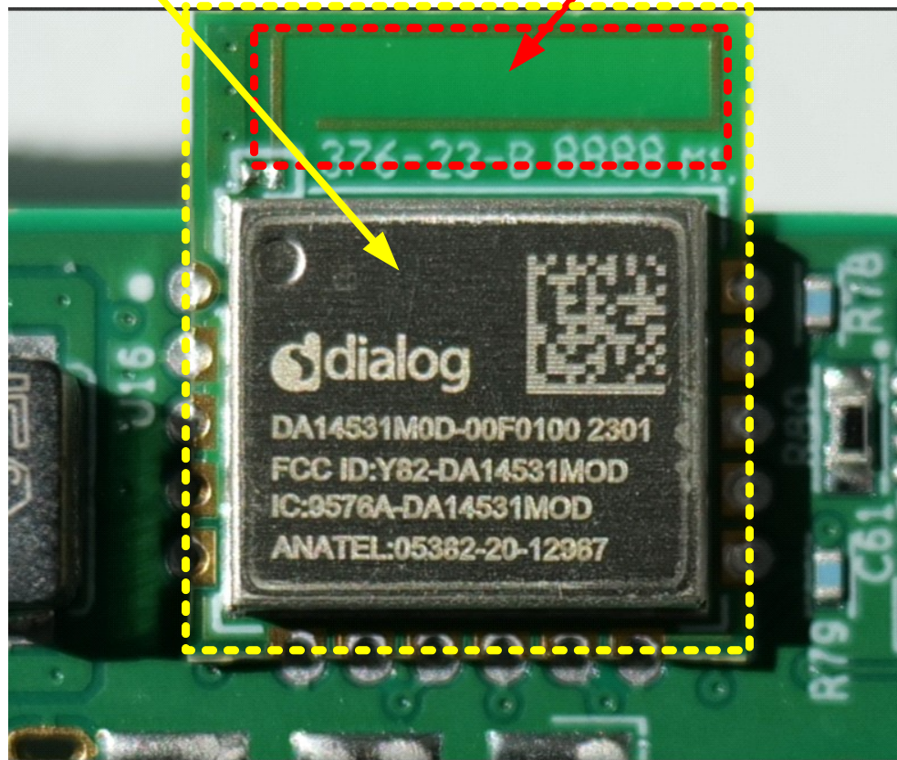
ZOOM IN OF BLE MODULE CIRCUIT
