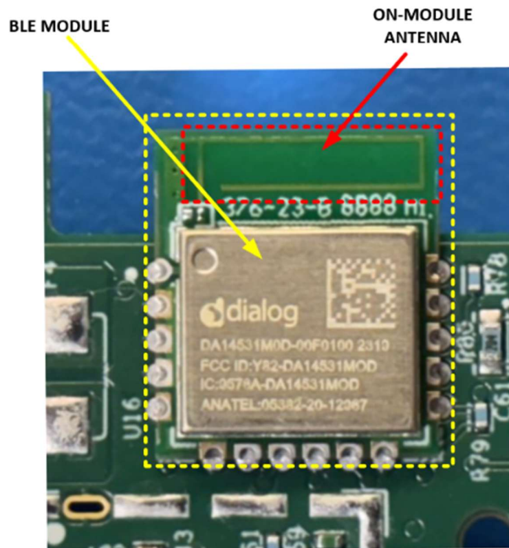
ZOOM IN OF BLE MODULE CIRCUIT
