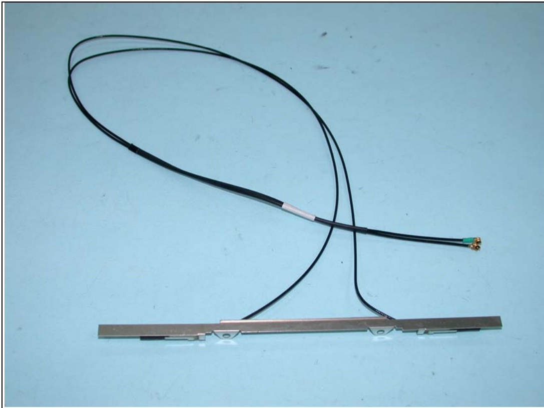
( Antenna Model No.: EW1B)
