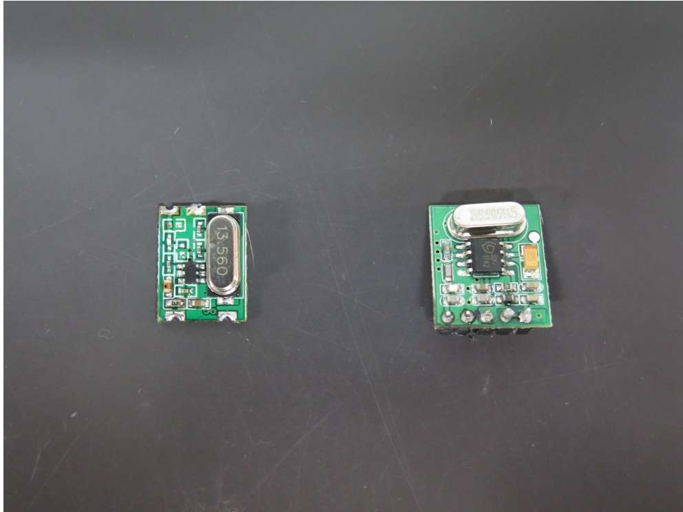
LQ-803 TX AND RX MODULE
