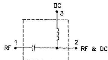
Bias-T Functionality
