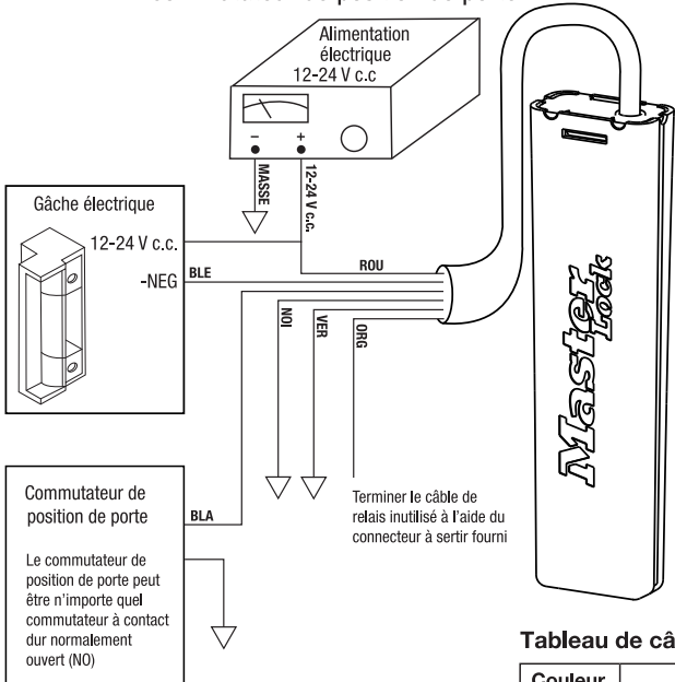
Schéma 2 : Câblage pour gâche électrique avec commutateur de position de porte
