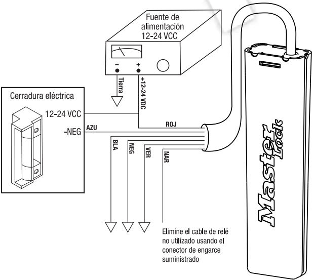
Diagrama 1: Cableado para cerradura eléctrica
