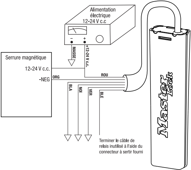
Schéma 3 : Câblage pour serrure magnétique
