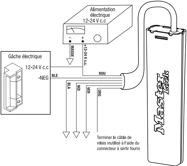
Schéma 1 : Câblage pour gâche électrique
