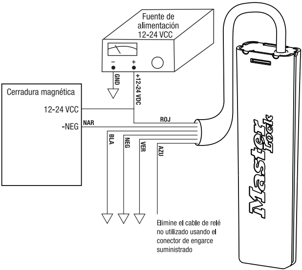
Diagrama 3: Cableado para cerradura magnética
