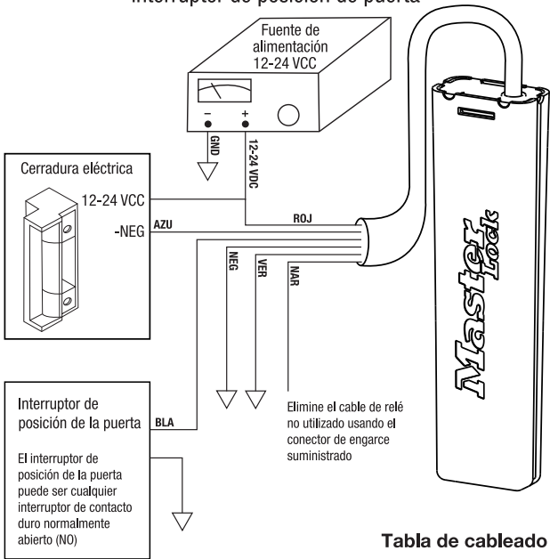
Diagrama 2: Cableado para cerradura eléctrica con interruptor de posición de puerta
