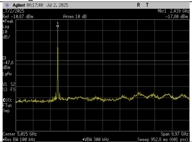
Mid Ch_2440MHz_10MHz BW_-30dBc_30MHz-10GHz_Port 2
