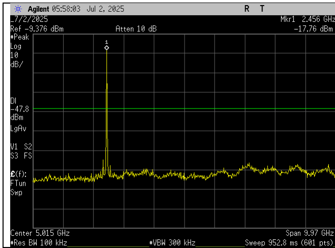
High Ch_2457MHz_10MHz BW_-30dBc_30MHz-10GHz_Port 1
