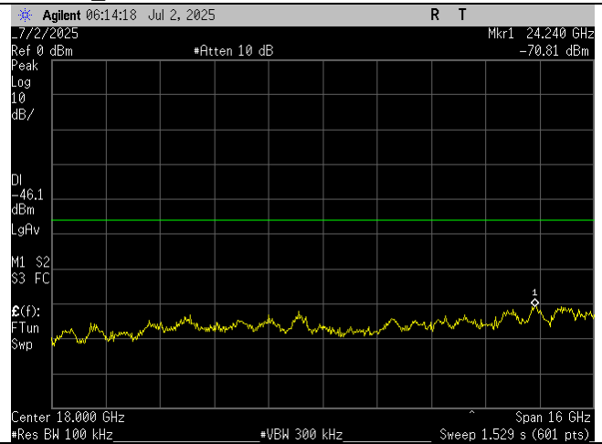
Low Ch_2418MHz_10MHz BW_-30dBc_10-26GHz_Port 2
