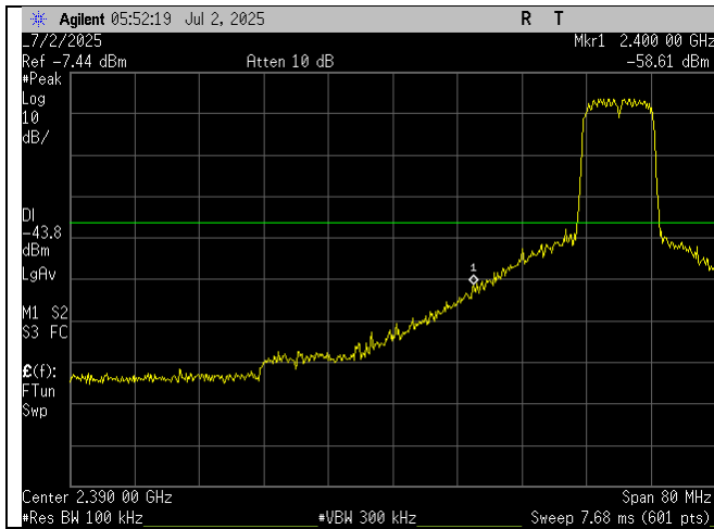
Low Ch_2418MHz_10MHz BW_-30dBc_Lower Band Edge_Port 1
