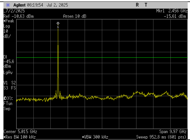
High Ch_2457MHz_10MHz BW_-30dBc_30MHz-10GHz_Port 2
