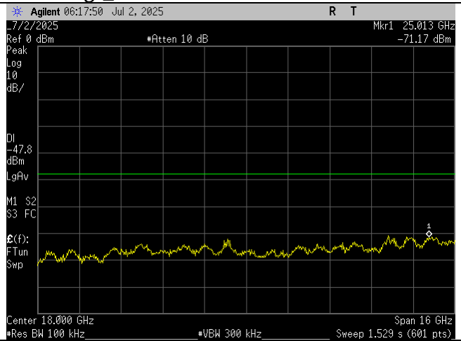
Mid Ch_2440MHz_10MHz BW_-30dBc_10-26GHz_Port 2
