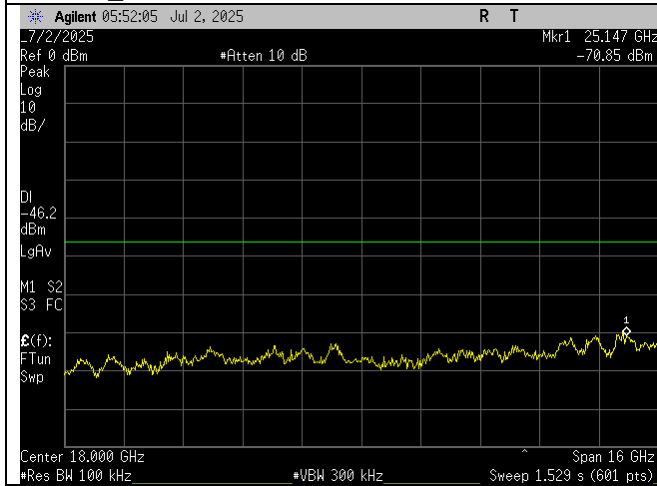
Low Ch_2418MHz_10MHz BW_-30dBc_10-26GHz_Port 1
