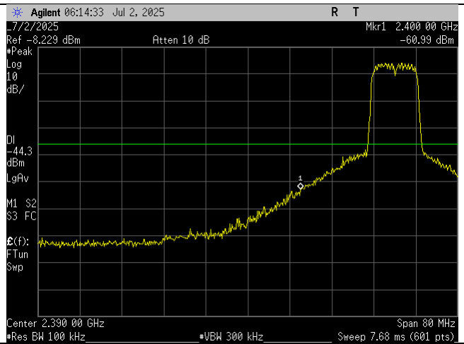
Low Ch_2418MHz_10MHz BW_-30dBc_Lower Band Edge_Port 2
