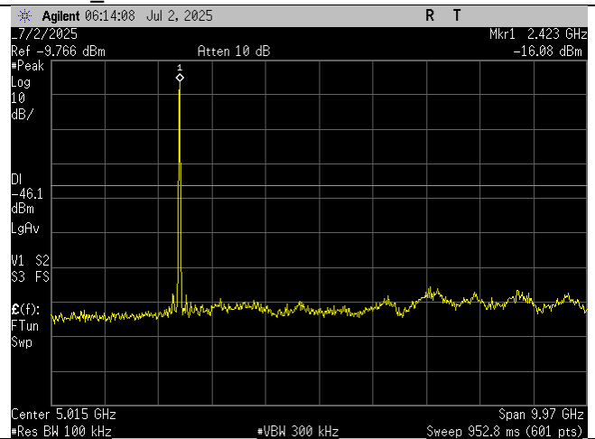
Low Ch_2418MHz_10MHz BW_-30dBc_30MHz-10GHz_Port 2
