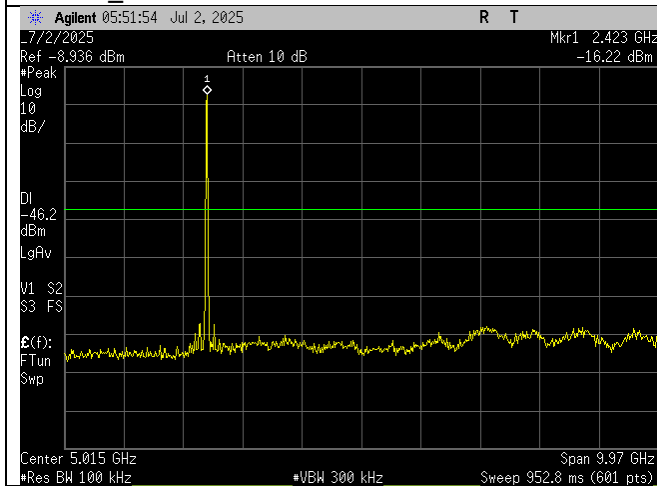
Low Ch_2418MHz_10MHz BW_-30dBc_30MHz-10GHz_Port 1
