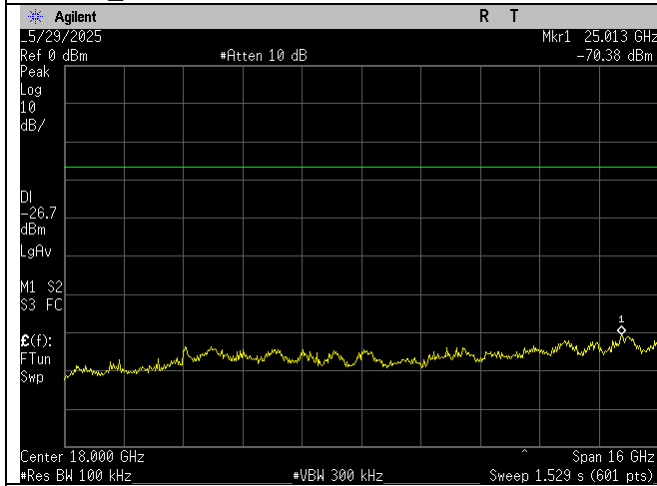
Low Ch_2416MHz_10MHz BW_-30dBc_10-26GHz_Port 1
