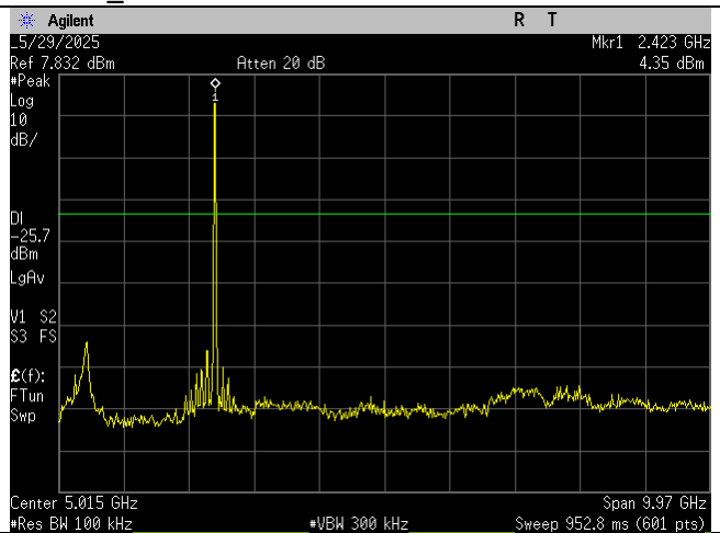
Low Ch_2416MHz_10MHz BW_-30dBc_30MHz-10GHz_Port 2
