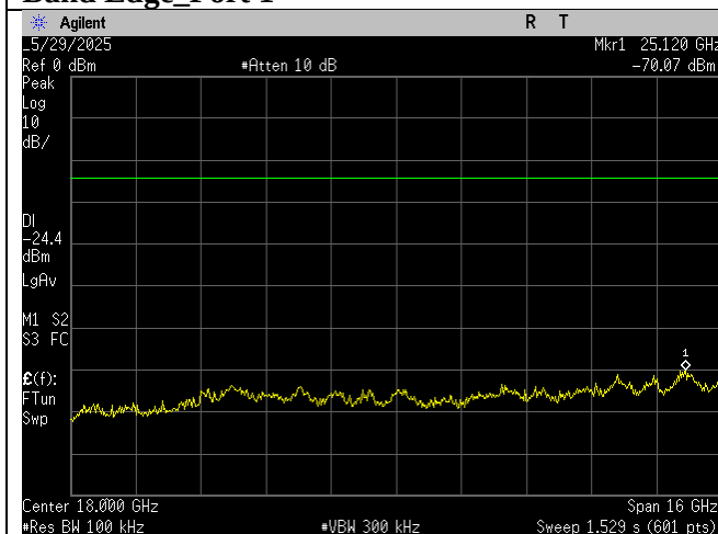
High Ch_2457MHz_10MHz BW_-30dBc_10-26GHz_Port 1
