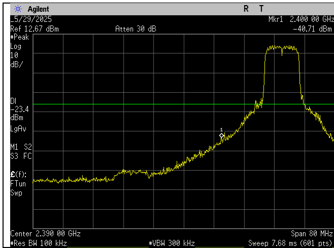
Low Ch_2416MHz_10MHz BW_-30dBc_Lower Band Edge_Port 1
