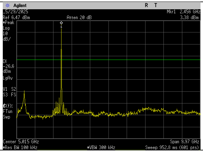
High Ch_2457MHz_10MHz BW_-30dBc_30MHz-10GHz_Port 2
