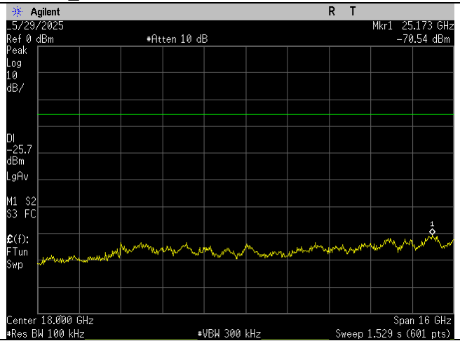
Low Ch_2416MHz_10MHz BW_-30dBc_10-26GHz_Port 2
