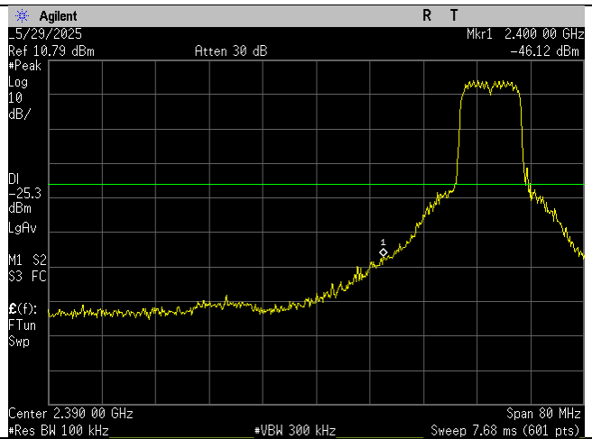
Low Ch_2416MHz_10MHz BW_-30dBc_Lower Band Edge_Port 2
