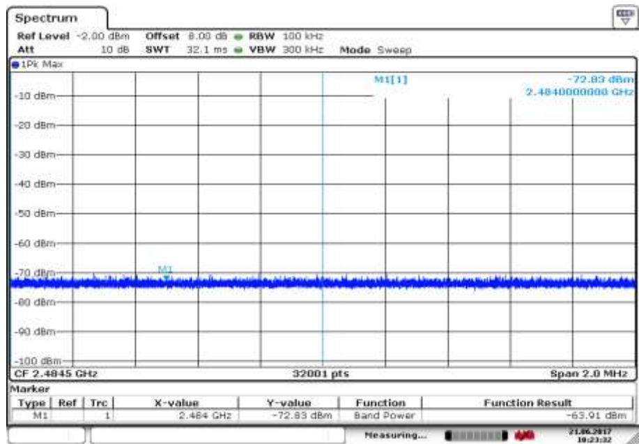
Plot 2: Upper band edge
