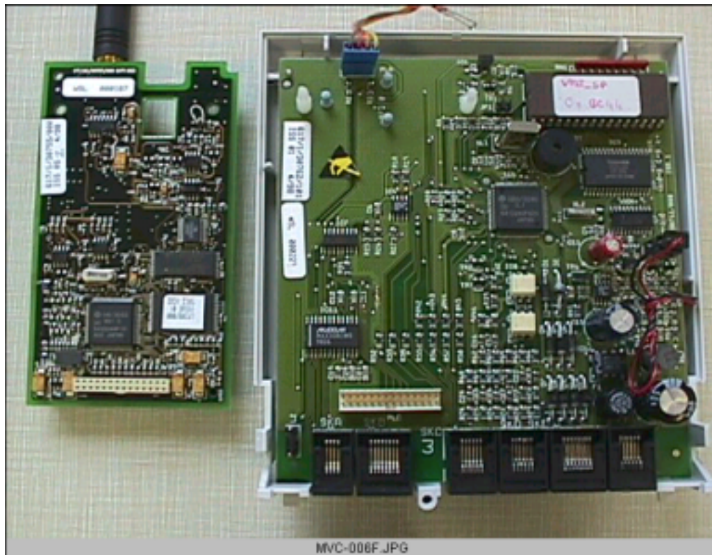
GPT Modem - RF PCB and VIU PCB
