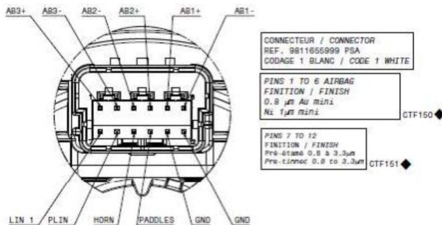
Détail T
