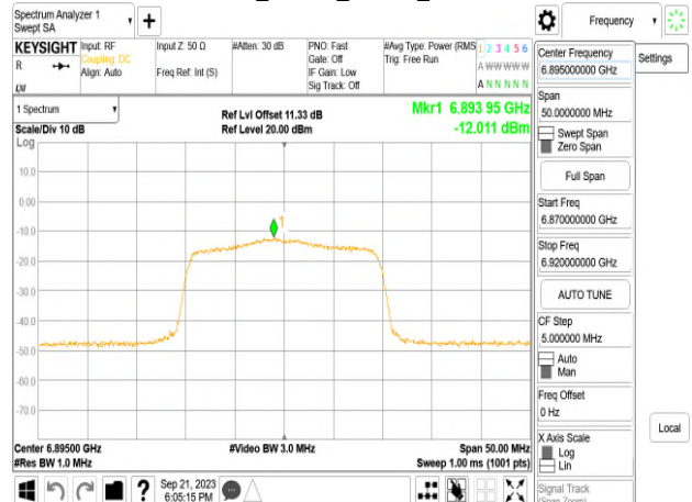
802.11a_20MHz_Chain1_6895MHz
