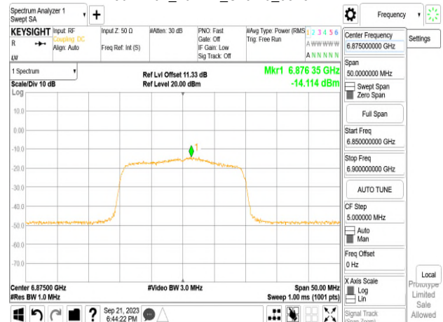
802.11ax_20MHz_Chain0_6875MHz
