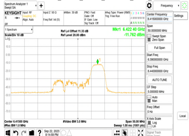
802.11ax_20MHz_Chain1_6415MHz_RU52_40
