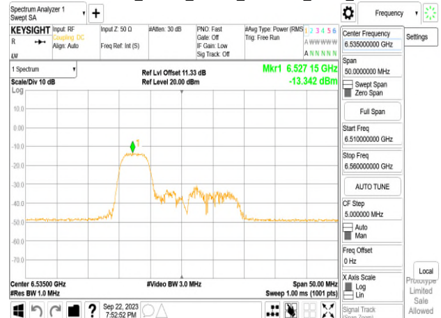
802.11ax_20MHz_Chain0_6535MHz_RU52_37
