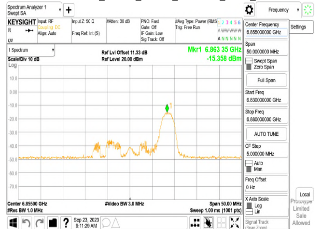
802.11ax_20MHz_Chain0_6855MHz_RU52_40
