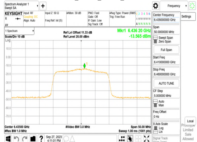
802.11ax_20MHz_Chain0_6435MHz
