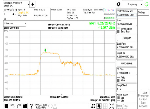
802.11ax_20MHz_Chain0_6535MHz_RU26_0
