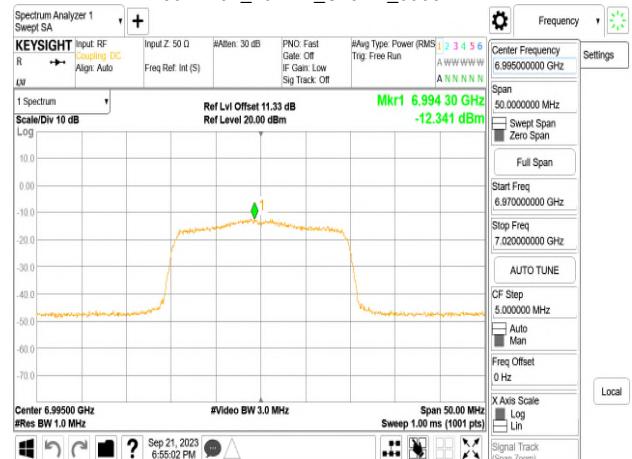
802.11ax_20MHz_Chain1_6995MHz
