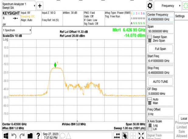
802.11ax_20MHz_Chain0_6435MHz_RU52_37
