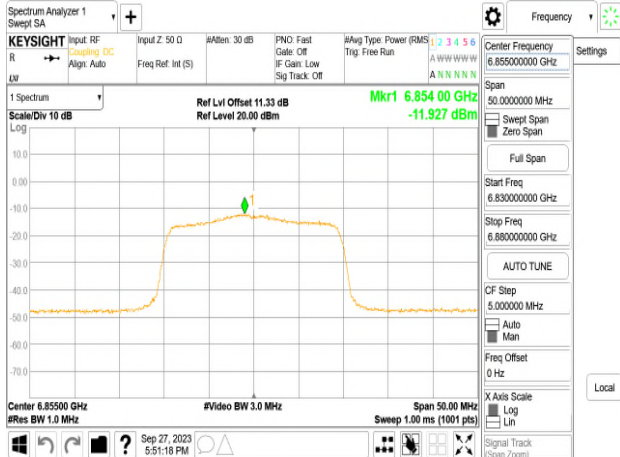
802.11ax_20MHz_Chain1_6855MHz
