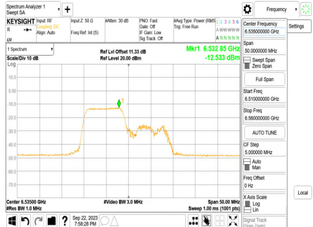
802.11ax_20MHz_Chain1_6535MHz_RU26_0
