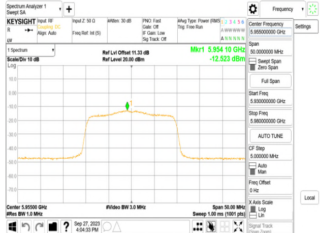
802.11ax_20MHz_Chain1_5955MHz_RU53
