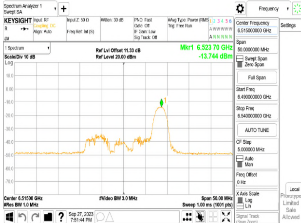
802.11ax_20MHz_Chain0_6515MHz_RU52_40
