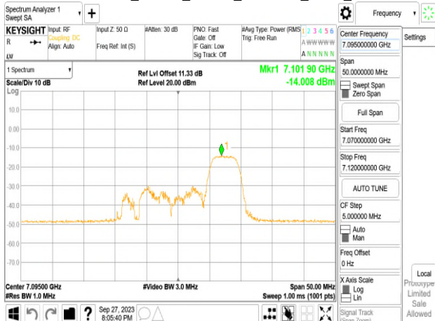
802.11ax_20MHz_Chain0_7095MHz_RU52_40
