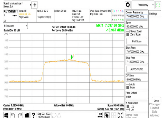
802.11ax_20MHz_Chain0_7095MHz
