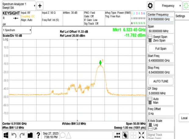
802.11ax_20MHz_Chain1_6515MHz_RU52_40
