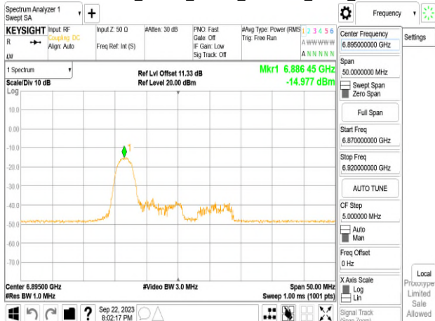
802.11ax_20MHz_Chain0_6895MHz_RU26_0
