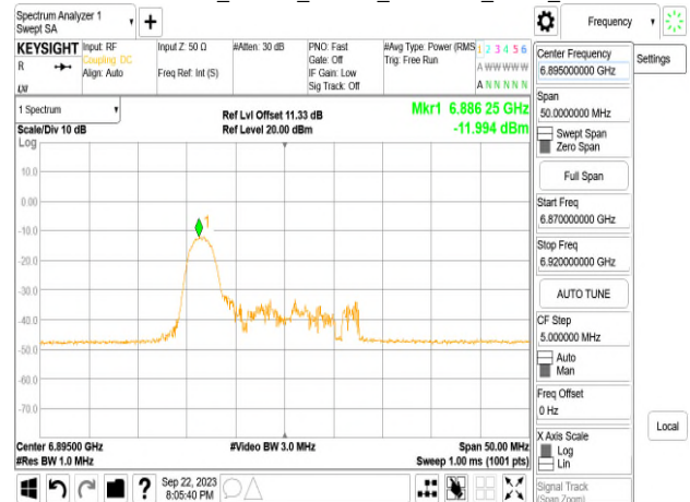
802.11ax_20MHz_Chain1_6895MHz_RU52_37
