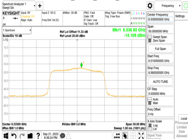
802.11ax_20MHz_Chain0_6535MHz
