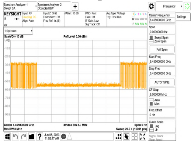
802.11ax_20MHz_CF 6455MHz_Interference_6455MHz_ -74.6dBm_Minimal
