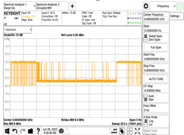
802.11ax_160MHz_CF 6665MHz_Interference_6665MHz_-72.16dBm_Normal
