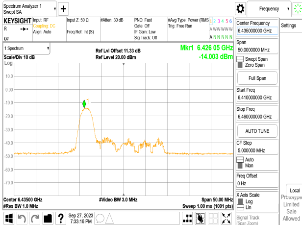
802.11ax_20MHz_Chain0_6435MHz_RU52_37
