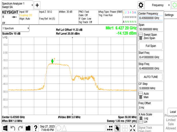
802.11ax_20MHz_Chain0_6435MHz_RU26_0
