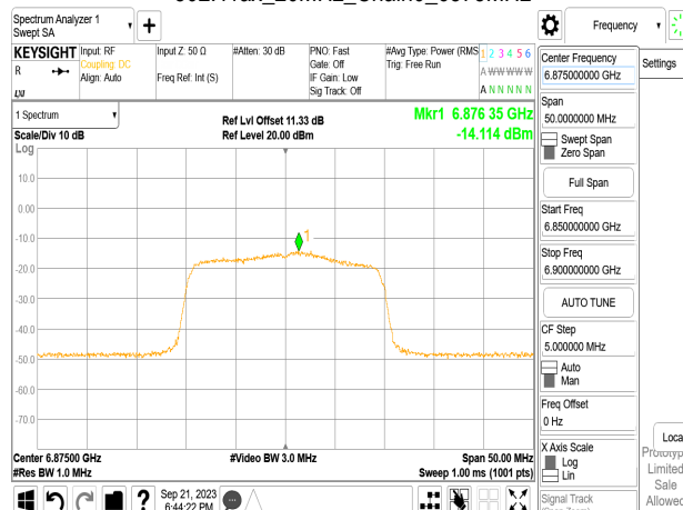
802.11ax_20MHz_Chain0_6875MHz
