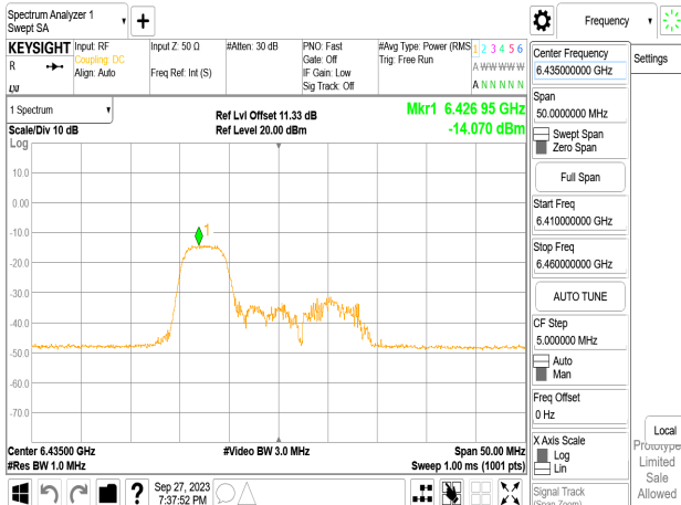
802.11ax_20MHz_Chain0_6435MHz_RU52_37
