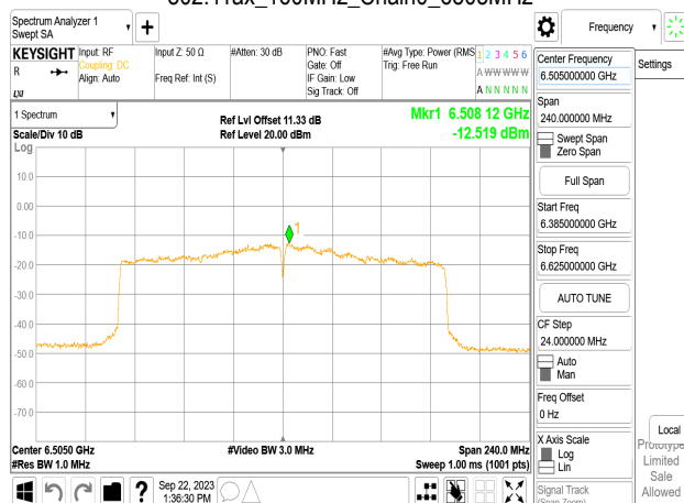
802.11ax_160MHz_Chain0_6505MHz
