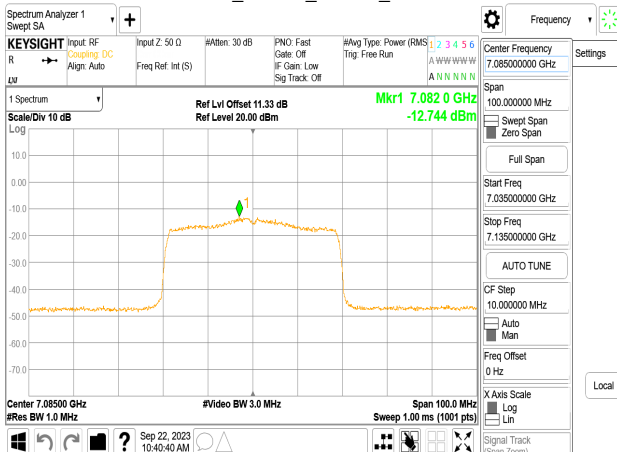
802.11ax_40MHz_Chain1_7085MHz
