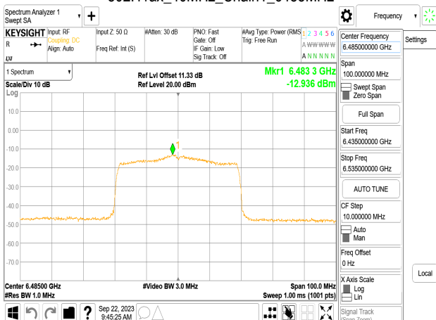
802.11ax_40MHz_Chain1_6485MHz
