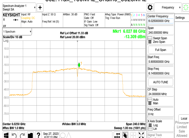
802.11ax_160MHz_Chain0_6025MHz_RU996_67
