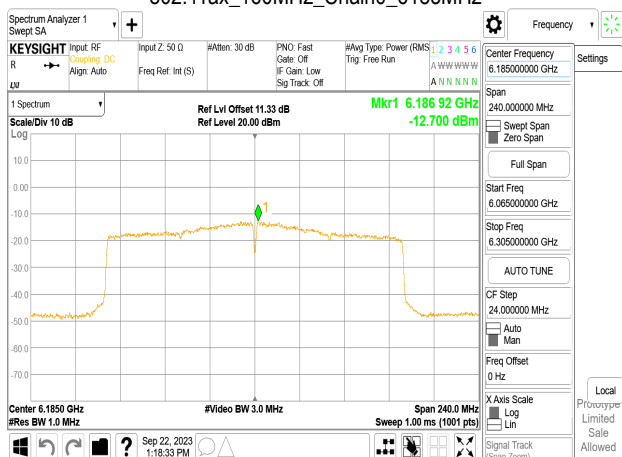
802.11ax_160MHz_Chain0_6185MHz
