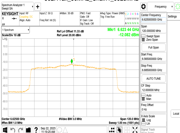
802.11ax_80MHz_Chain1_6625MHz
