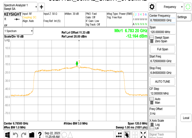
802.11ax_80MHz_Chain1_6785MHz
