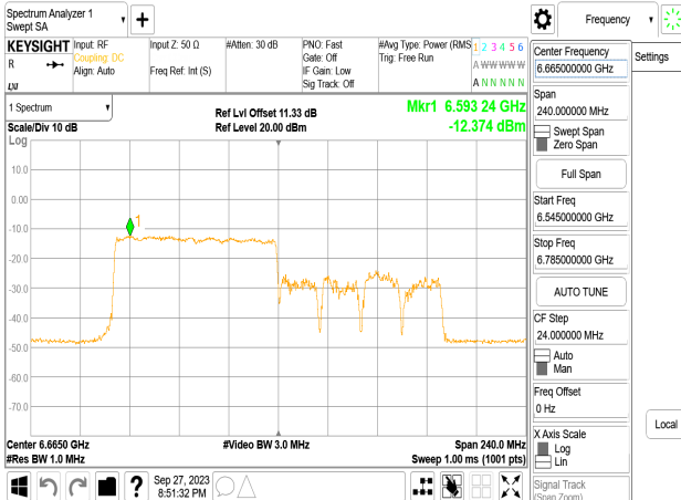
802.11ax_160MHz_Chain1_6665MHz_RU996_67
