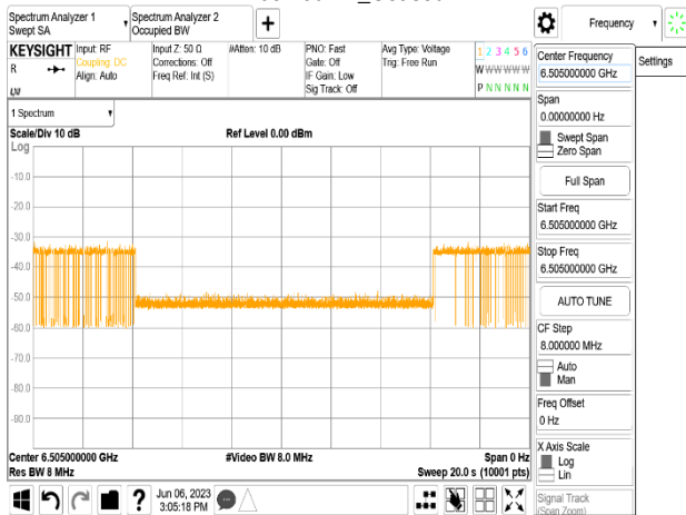
802.11ax_160MHz_CF 6505MHz_Interference_6505MHz_-67.46dBm_Minimal
