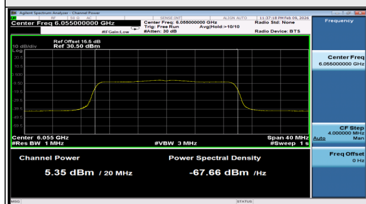
802.11be (EHT20) / CH21 Chain 0
