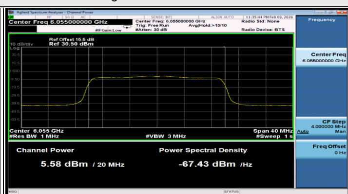
802.11be (EHT20) / CH21 Chain 1
