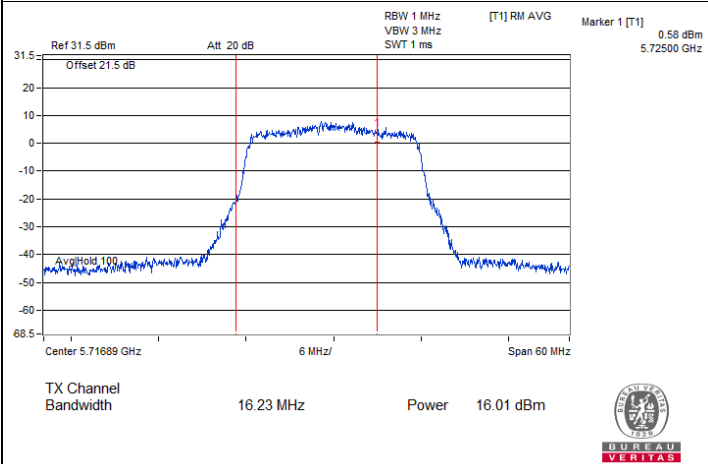
Chain 1 : CH 144 (U-NII-2C)
