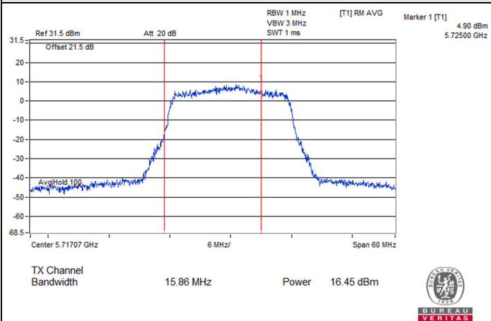
Chain 0 : CH 144 (U-NII-2C)
