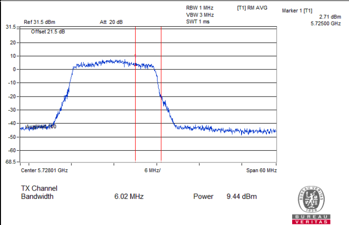
Chain 1 : CH 144 (U-NII-3)
