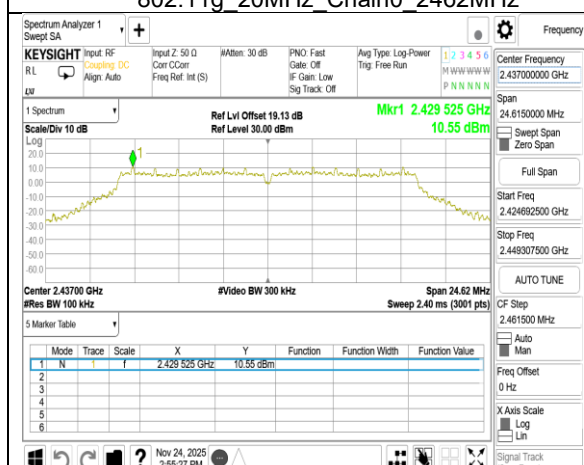
802.11g_20MHz_Chain1_2437MHz
