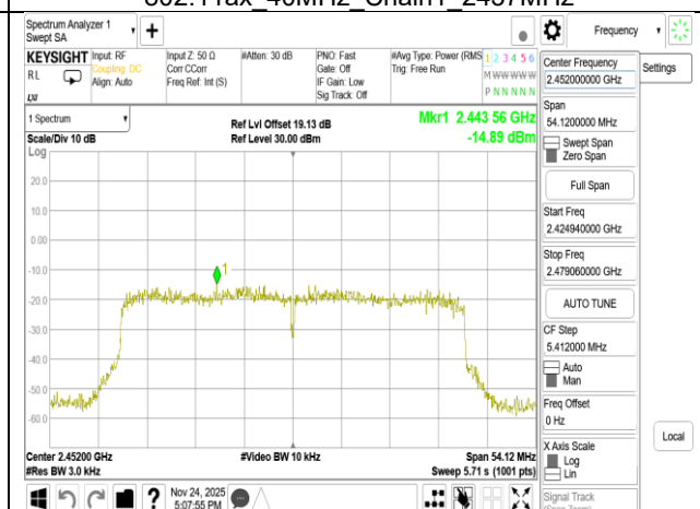
802.11ax_40MHz_Chain1_2452MHz
