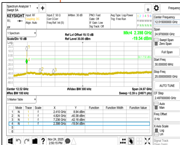
802.11g_20MHz_Chain0_2412MHz
