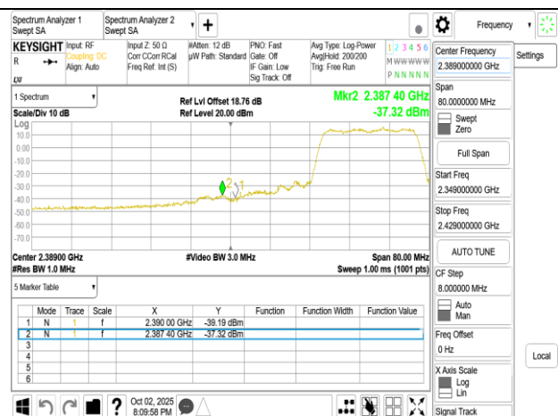
802.11ax 20MHz Chain1 2417MHz
