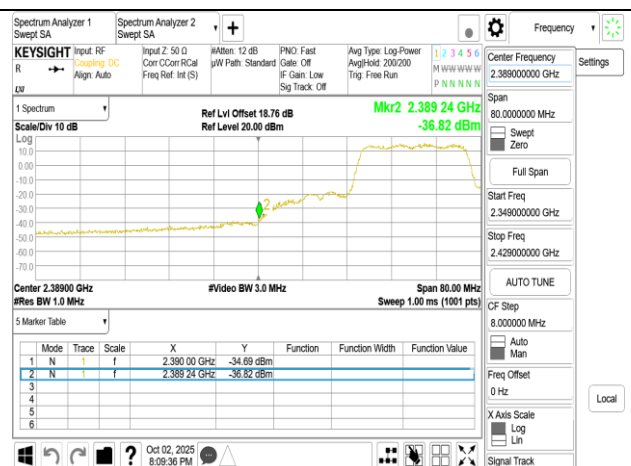
802.11ax_20MHz_Chain0_2417MHz
