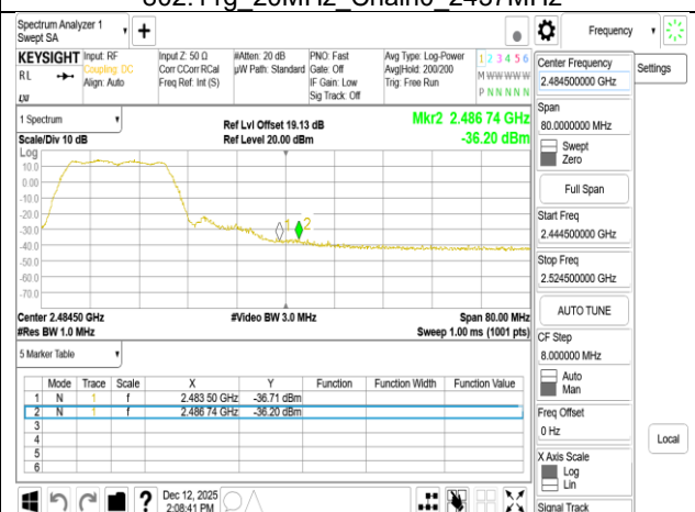
802.11g 20MHz Chain0 2457MHz
