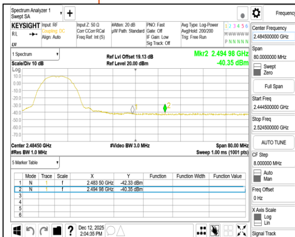
802.11b 20MHz Chain1 2457MHz
