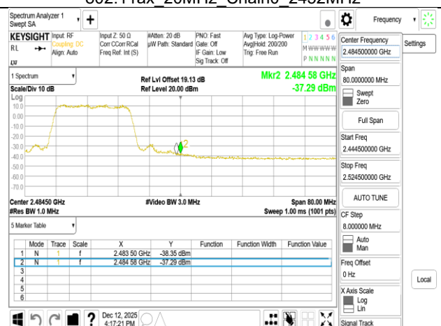
802.11ax_20MHz_Chain0_2462MHz
