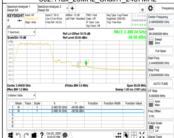
802.11ax 20MHz Chain1 2457MHz
