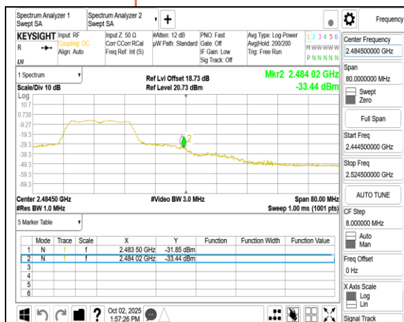
802.11g 20MHz Chain0 2462MHz
