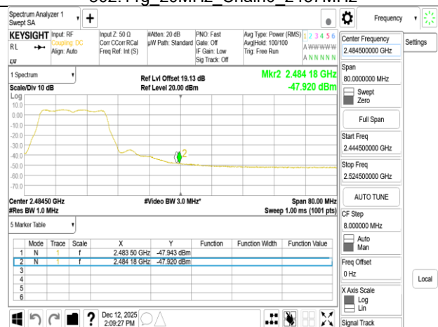
802.11g 20MHz Chain0 2457MHz
