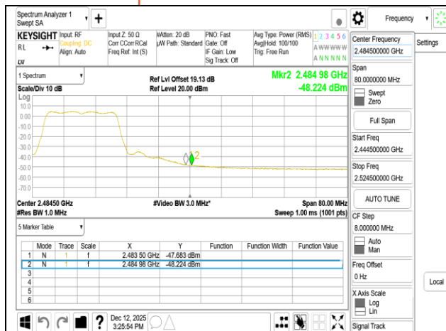
802.11n 20MHz Chain0 2457MHz
