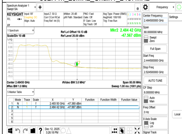
802.11n 20MHz Chain1 2457MHz
