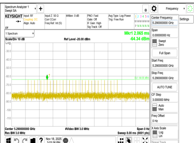
HE80_5290_Type 2.PNG
