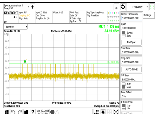
HE20_5500_Type 2.PNG
