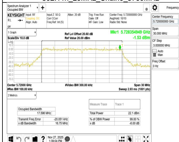
802.11n 20MHz Chain0_5720MHz UNII-3
