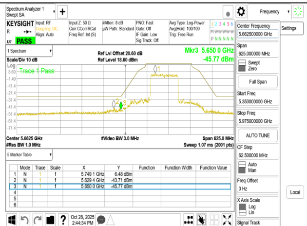
802.11ax_80MHz_Chain1_5775MHz
