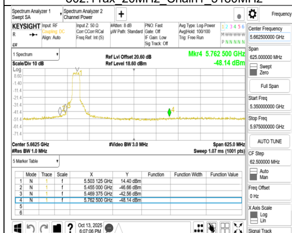
802.11ax 20MHz Chain1 5500MHz
