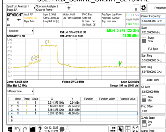
802.11ax 80MHz Chain1 5530MHz
