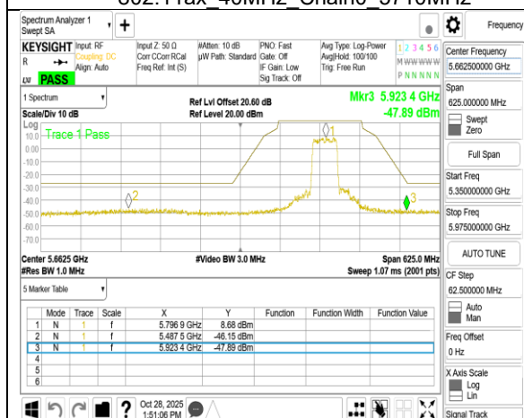
802.11ax 40MHz Chain0 5795MHz
