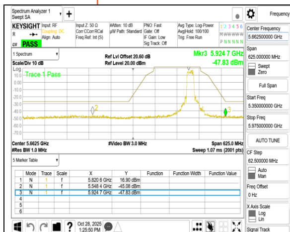
802.11ax 20MHz Chain0 5825MHz
