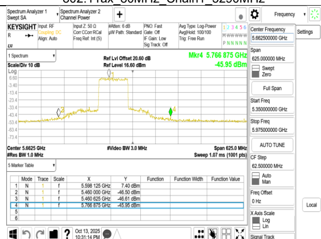
802.11ax 80MHz Chain1 5610MHz
