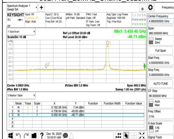
802.11ax 20MHz Chain1 5180MHz
