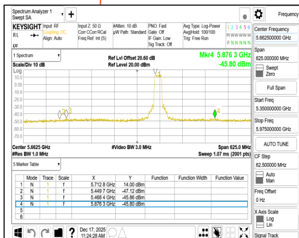
802.11ax 20MHz Chain1 5720MHz
