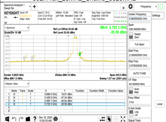
802.11ax 20MHz Chain0 5700MHz
