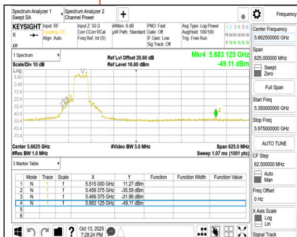
802.11ax 40MHz Chain0 5510MHz
