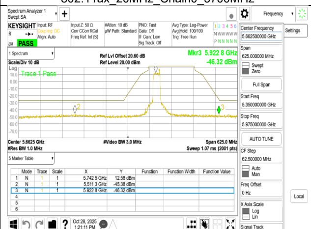
802.11ax 20MHz Chain0 5745MHz
