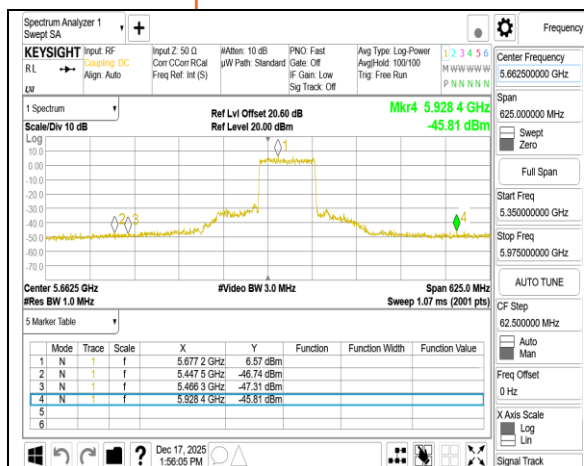
802.11ax 80MHz Chain0 5690MHz
