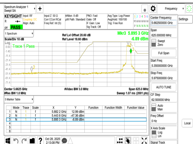
802.11ax 20MHz Chain0 5885MHz
