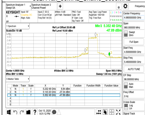
802.11ax 80MHz Chain1 5210MHz
