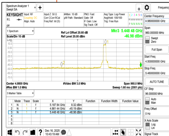
802.11ax 20MHz Chain0 5180MHz
