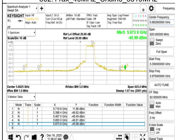
802.11ax 40MHz Chain0 5710MHz
