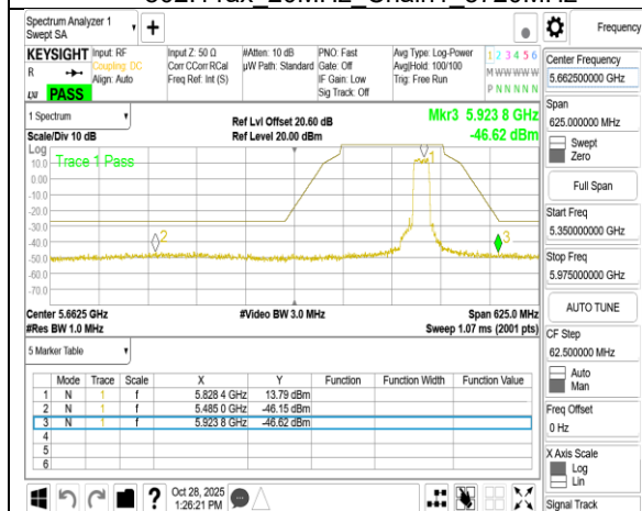
802.11ax 20MHz Chain1 5825MHz
