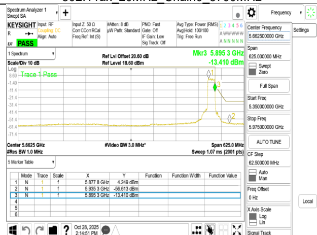
802.11ax 20MHz Chain0 5885MHz
