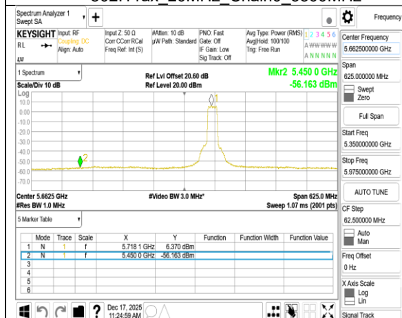
802.11ax 20MHz Chain0 5720MHz
