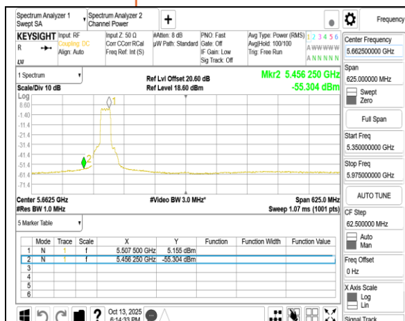
802.11ax 20MHz Chain0 5500MHz
