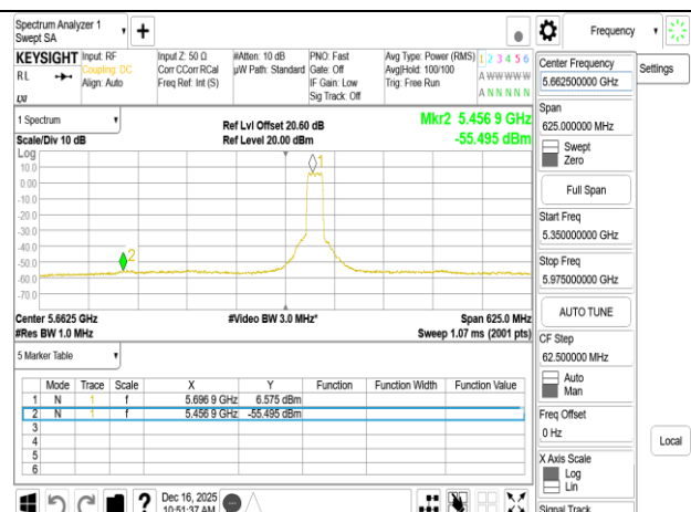
802.11ax 20MHz Chain0 5700MHz
