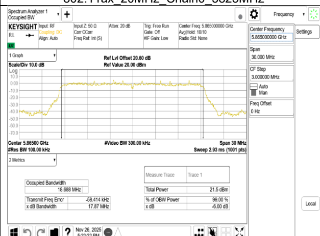
802.11ax 20MHz Chain0 5865MHz
