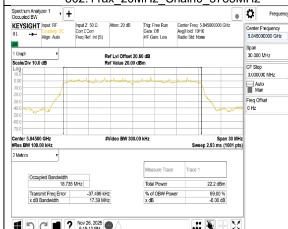
802.11ax 20MHz Chain0 5845MHz
