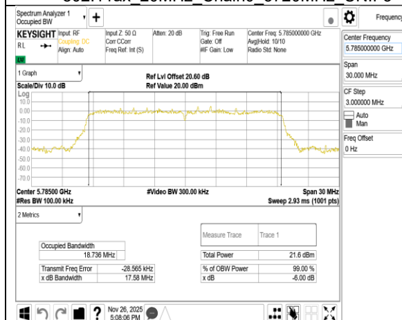
802.11ax 20MHz Chain0 5785MHz
