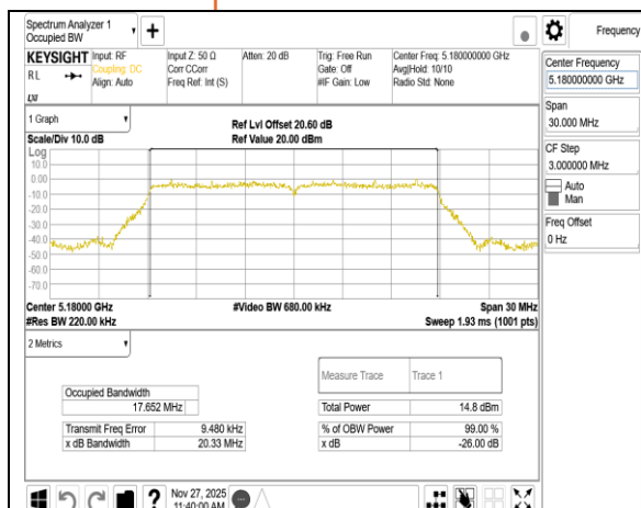
802.11n 20MHz Chain1 5180MHz
