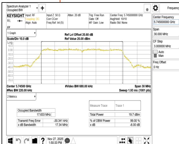
802.11n 20MHz Chain0_5745MHz
