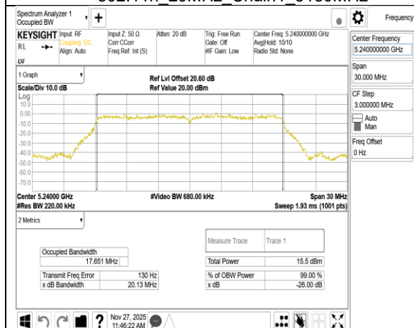
802.11n 20MHz Chain1 5240MHz
