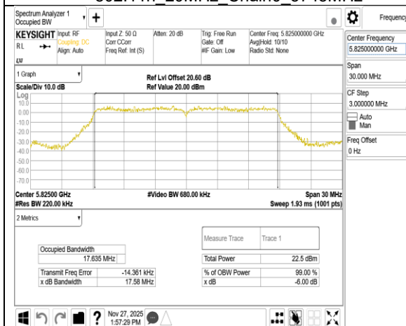
802.11n 20MHz Chain0_5825MHz
