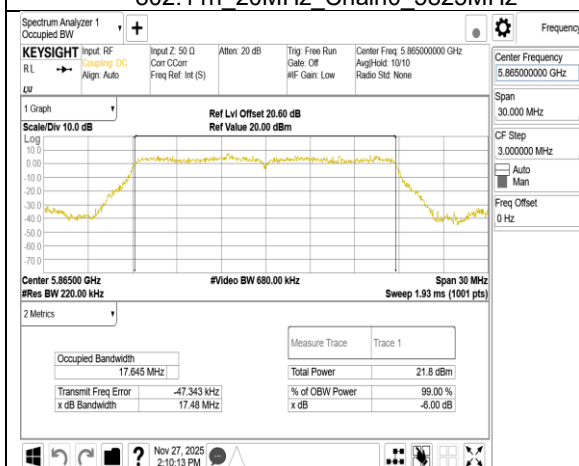
802.11n 20MHz Chain0_5865MHz
