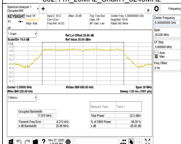
802.11n 20MHz Chain1 5300MHz
