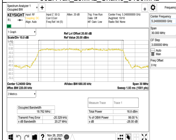
802.11ax 20MHz Chain0 5240MHz
