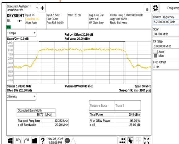
802.11ax 20MHz Chain1 5700MHz
