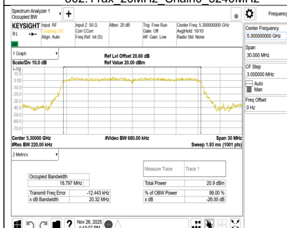
802.11ax 20MHz Chain0 5300MHz
