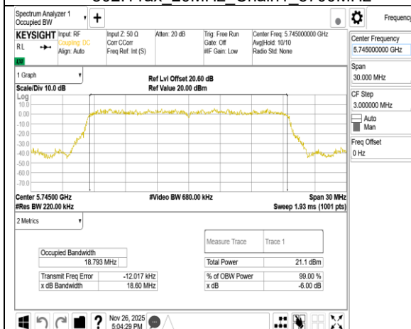
802.11ax 20MHz Chain1 5745MHz
