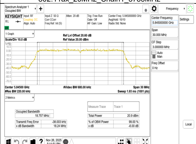
802.11ax 20MHz Chain1 5845MHz
