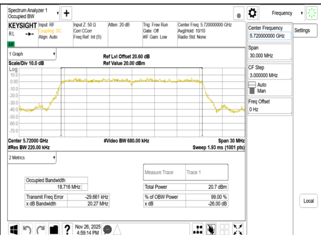
802.11ax 20MHz Chain1 5720MHz
