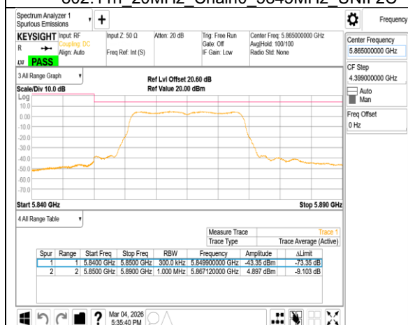
802.11n_20MHz_Chain0_5865MHz
