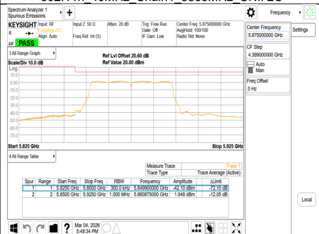
802.11n 40MHz Chain1 5875MHz
