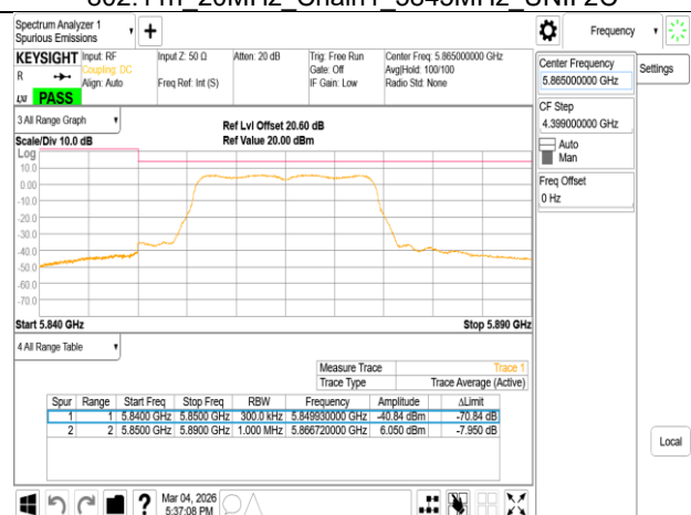
802.11n_20MHz_Chain1_5865MHz
