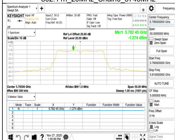
802.11n_20MHz_Chain0_5785MHz
