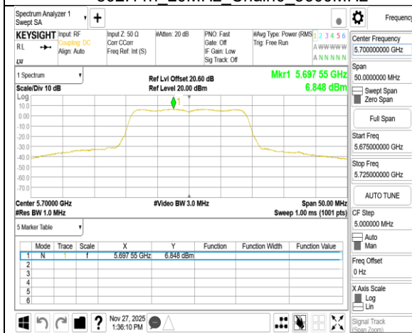
802.11n 20MHz Chain0_ 5700MHz
