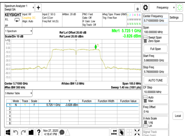
802.11n 40MHz Chain1 5710MHz UNII 3
