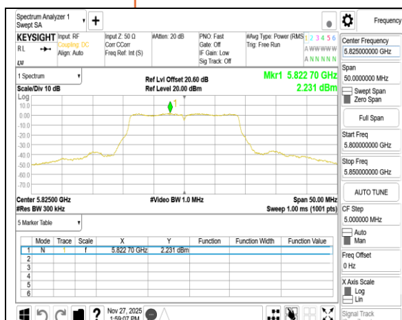
802.11n_20MHz_Chain0_5825MHz
