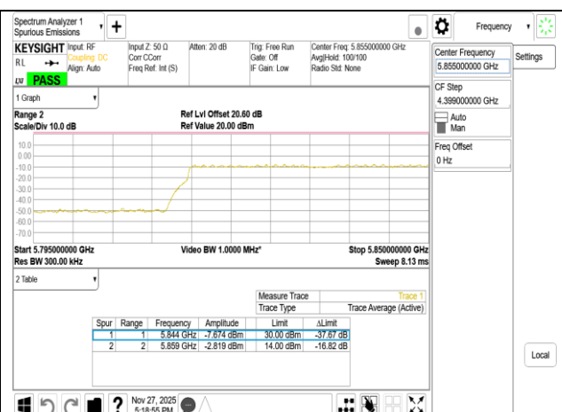
802.11ac 80MHz Chain1 5855MHz UNII 2C
