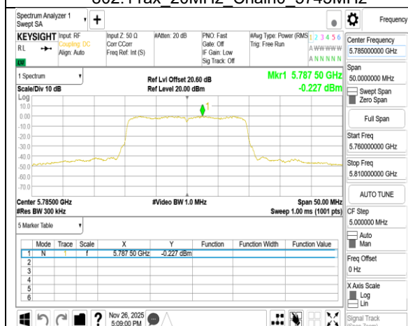
802.11ax_20MHz_Chain0_5785MHz
