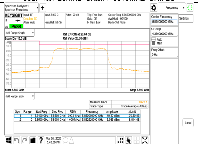
802.11ax 20MHz Chain1 5865MHz
