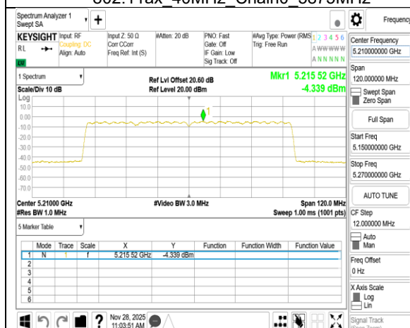
802.11ax_80MHz_Chain0_5210MHz
