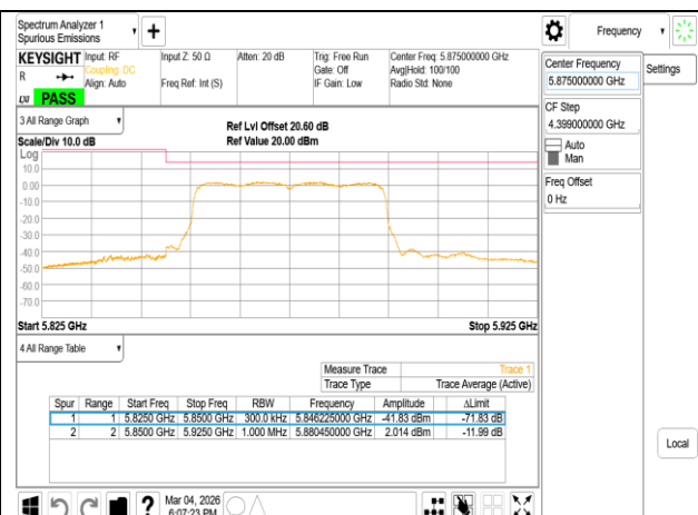
802.11ax_40MHz_Chain1_5875MHz
