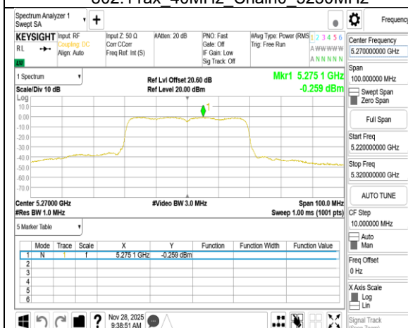
802.11ax 40MHz Chain0 5270MHz
