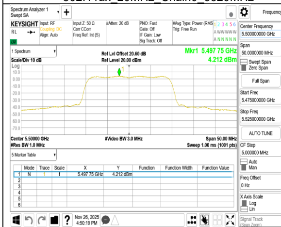
802.11ax 20MHz Chain0 5500MHz
