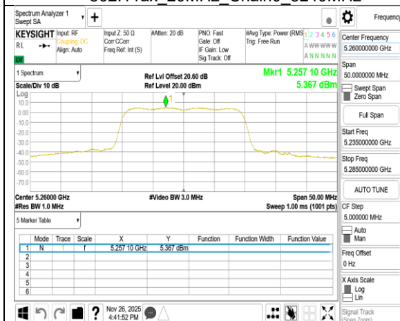
802.11ax 20MHz Chain0 5260MHz
