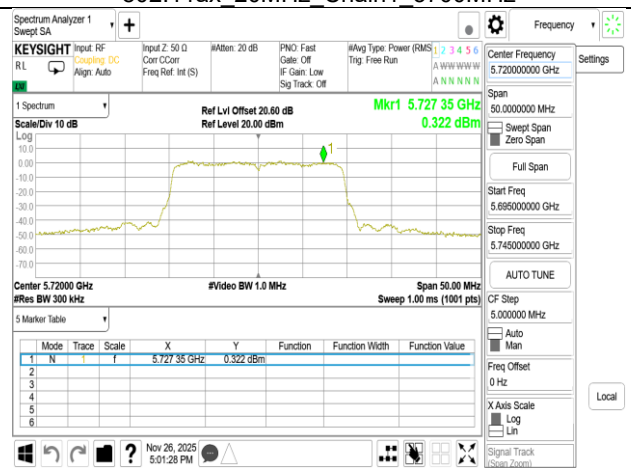
802.11ax 20MHz Chain0 5720MHz UNII 3
