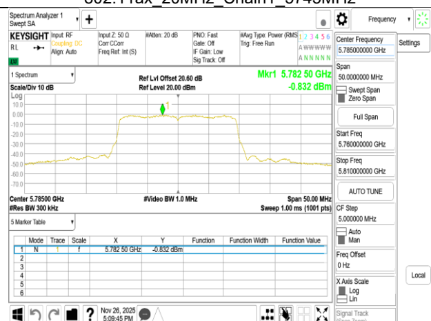
802.11ax_20MHz_Chain1_5785MHz
