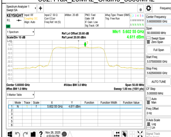
802.11ax 20MHz Chain0 5600MHz
