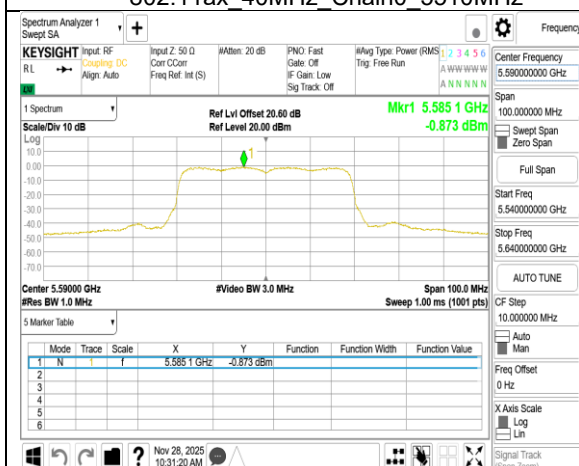
802.11ax 40MHz Chain0 5590MHz
