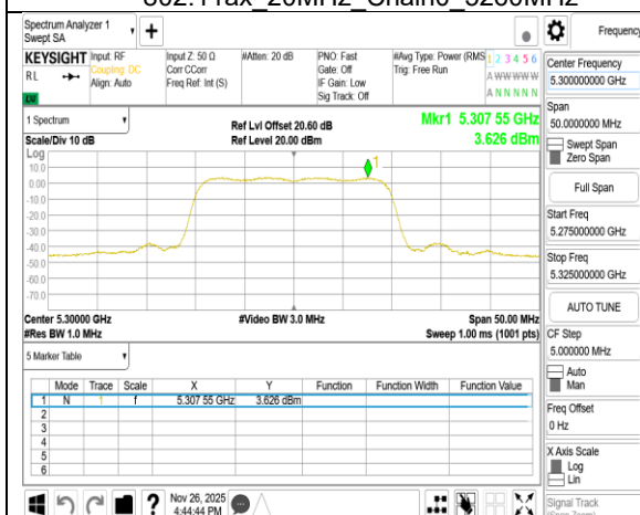
802.11ax 20MHz Chain0 5300MHz
