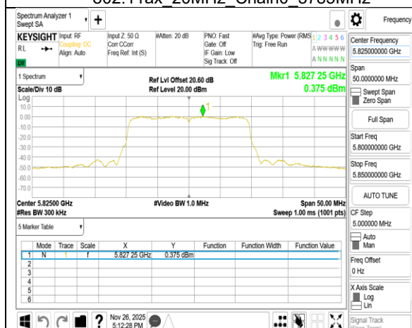
802.11ax_20MHz_Chain0_5825MHz
