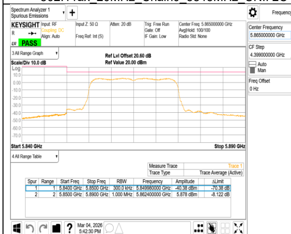
802.11ax 20MHz Chain0 5865MHz
