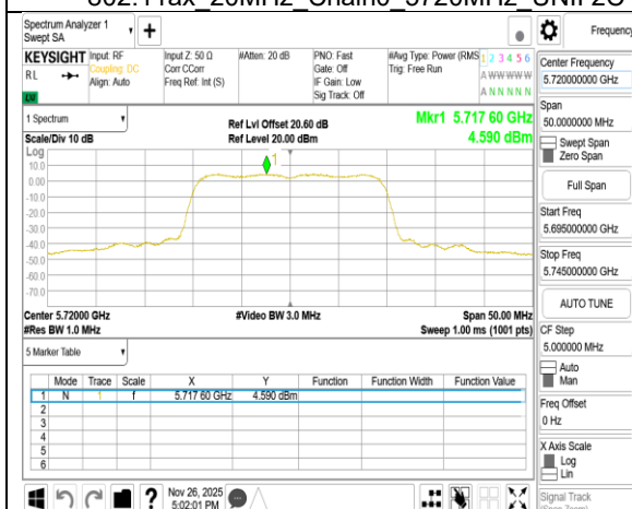
802.11ax 20MHz Chain1 5720MHz UNII 2C
