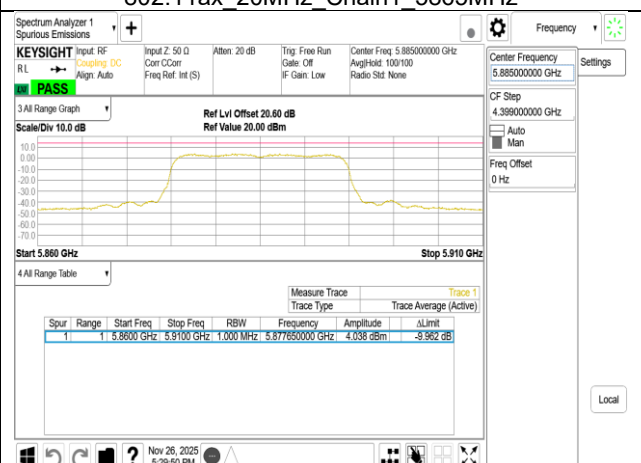
802.11ax 20MHz Chain1 5885MHz
