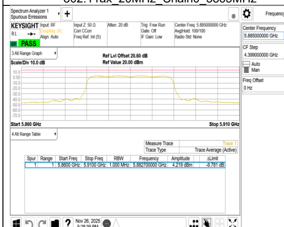
802.11ax 20MHz Chain0 5885MHz
