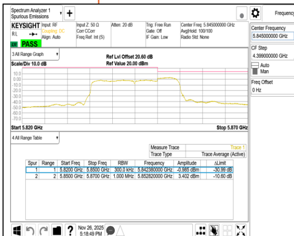
802.11ax 20MHz Chain0 5845MHz UNII 2C
