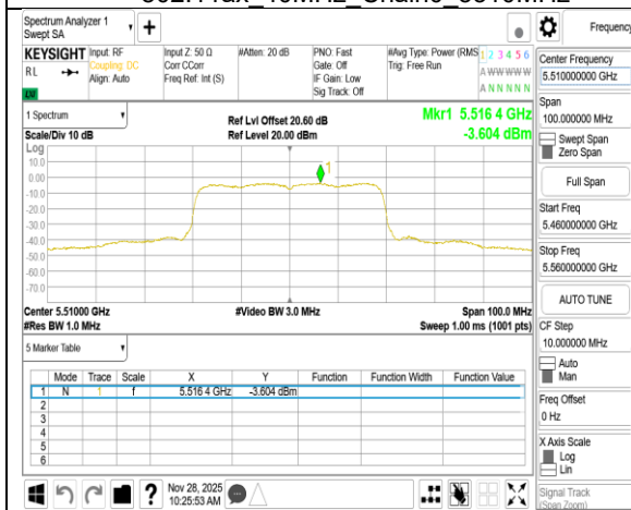
802.11ax 40MHz Chain0 5510MHz
