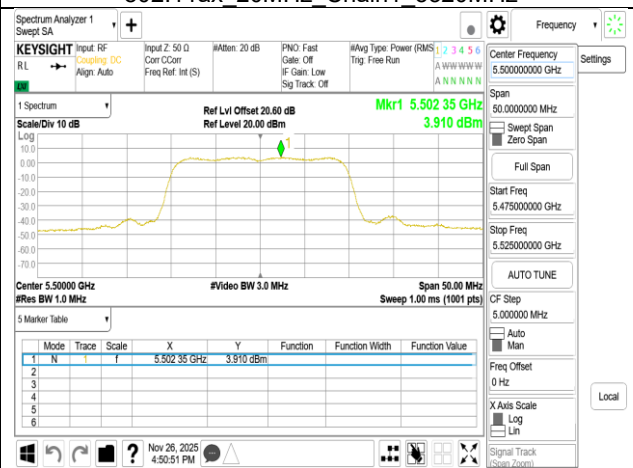
802.11ax 20MHz Chain1 5500MHz
