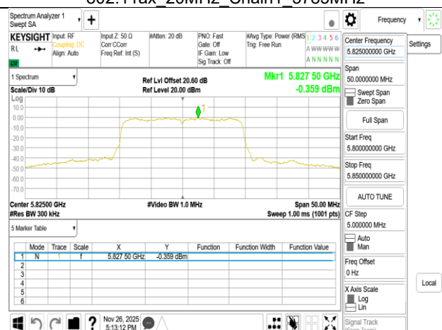
802.11ax_20MHz_Chain1_5825MHz
