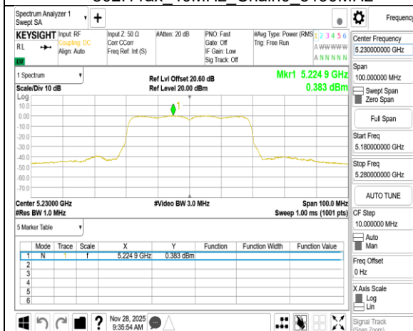
802.11ax 40MHz Chain0 5230MHz
