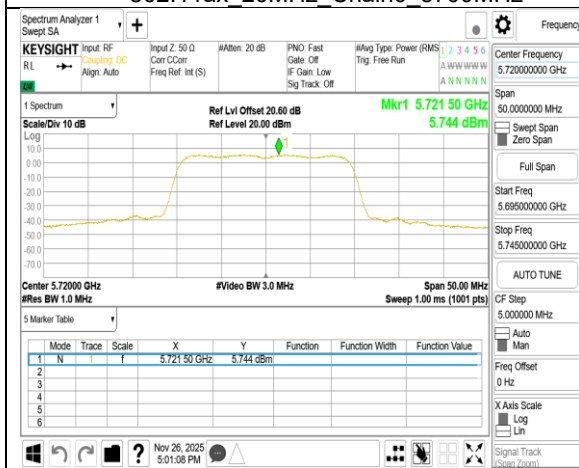
802.11ax 20MHz Chain0 5720MHz UNII 2C
