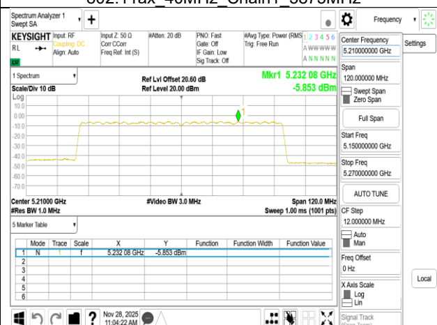
802.11ax_80MHz_Chain1_5210MHz
