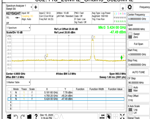
802.11a 20MHz Chain1 5180MHz
