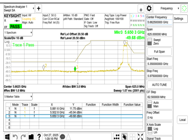
802.11a 20MHz Chain0 5885MHz
