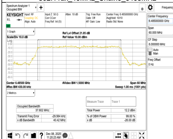
802.11ax 40MHz Chain0 6485MHz
