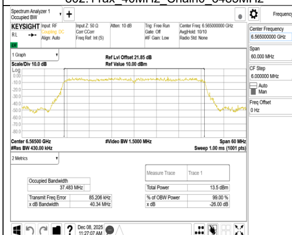
802.11ax 40MHz Chain0 6565MHz
