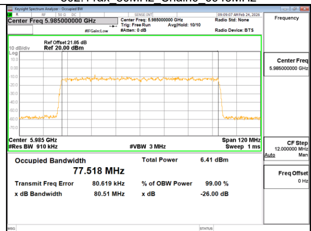
802.11ax 80MHz Chain1 5985MHz
