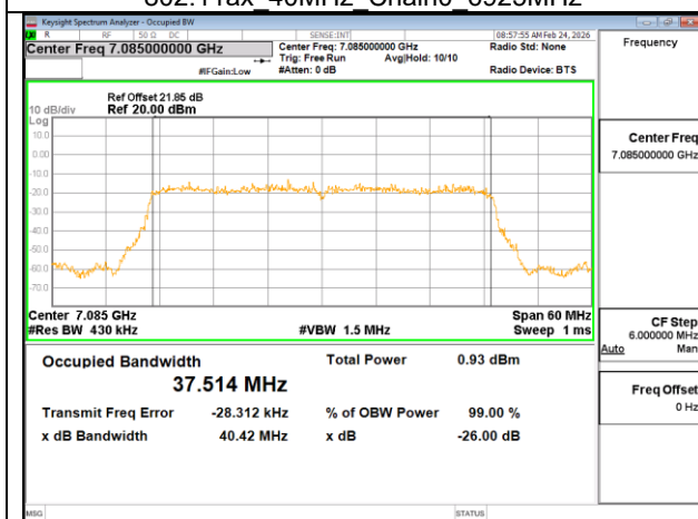
802.11ax 40MHz Chain0 7085MHz
