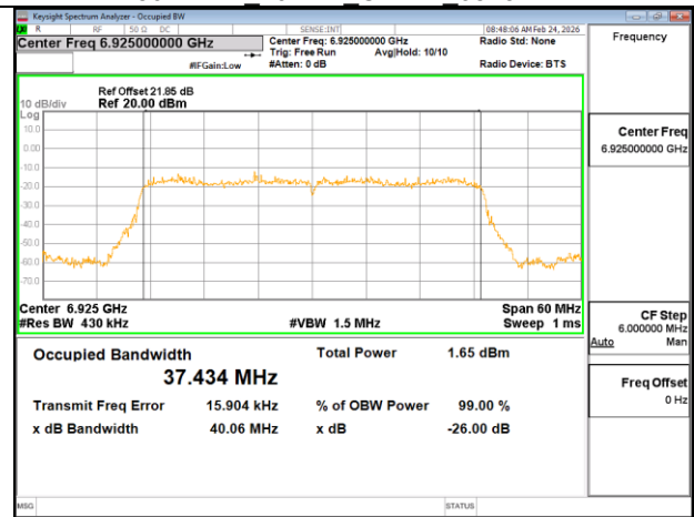
802.11ax 40MHz Chain1 6925MHz
