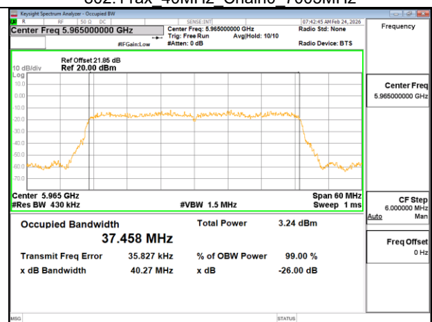
802.11ax 40MHz Chain1 5965MHz
