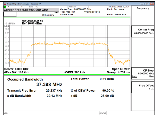
802.11ax 40MHz Chain0 6885MHz
