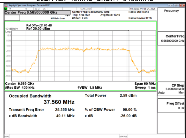
802.11ax 40MHz Chain1 6565MHz
