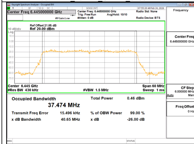
802.11ax 40MHz Chain1 6445MHz
