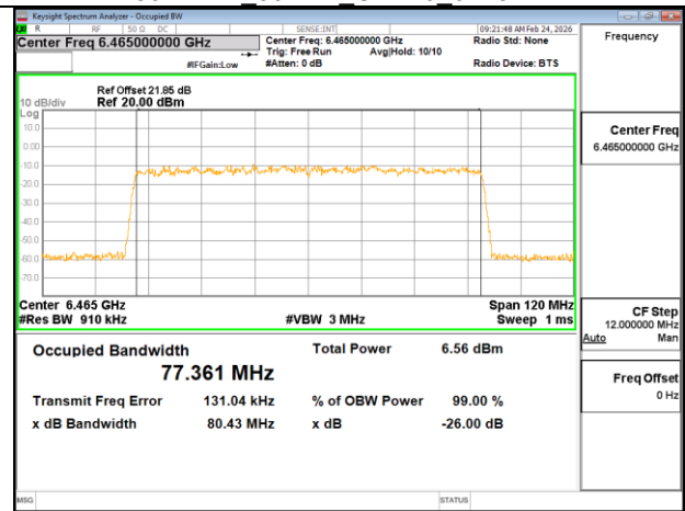
802.11ax 80MHz Chain0 6465MHz
