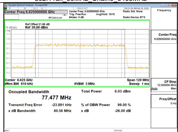
802.11ax 80MHz Chain0 6625MHz
