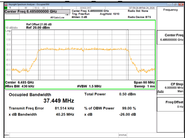
802.11ax 40MHz Chain1 6485MHz
