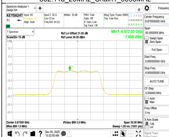
802.11a 20MHz Chain1 6875MHz
