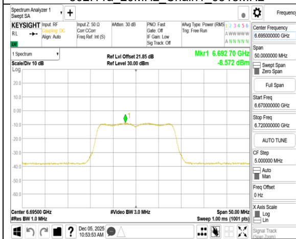
802.11a 20MHz Chain1 6695MHz
