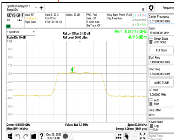
802.11a 20MHz Chain1 6515MHz
