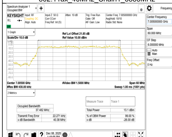
802.11ax 40MHz Chain1 7005MHz
