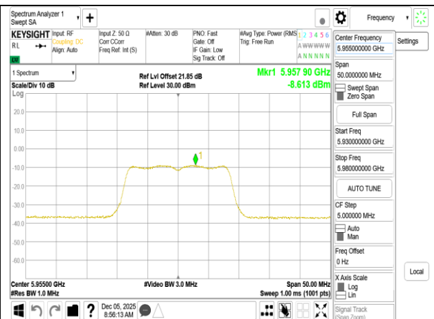
802.11a_20MHz_Chain1_5955MHz
