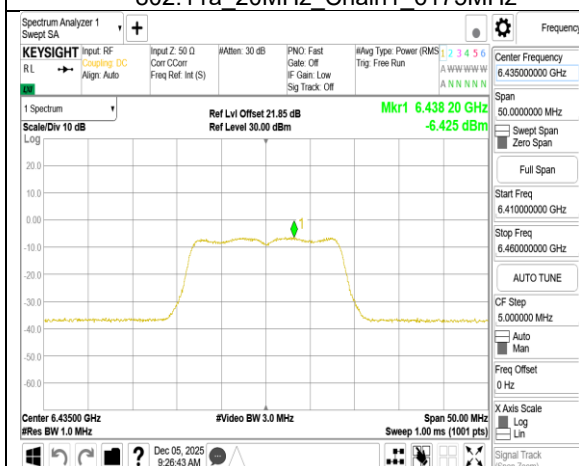
802.11a_20MHz_Chain1_6435MHz
